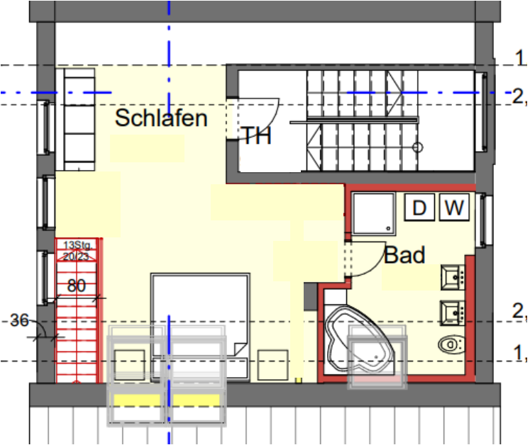
Grundriss DG
