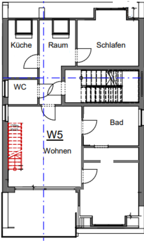
Grundriss 2. OG
