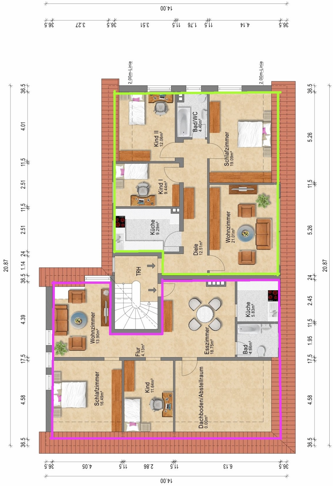
Dachgeschoss
