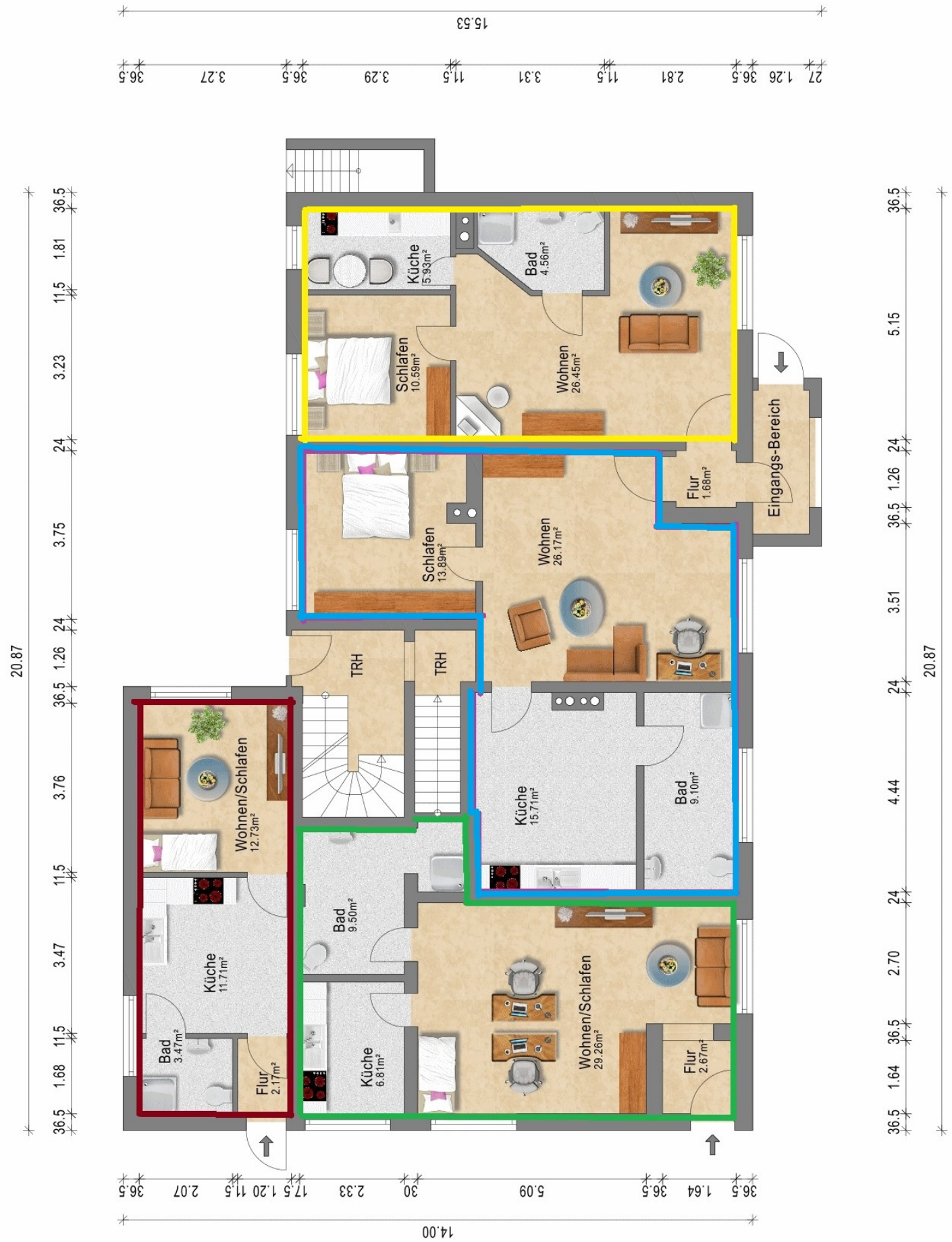
Erdgeschoss
