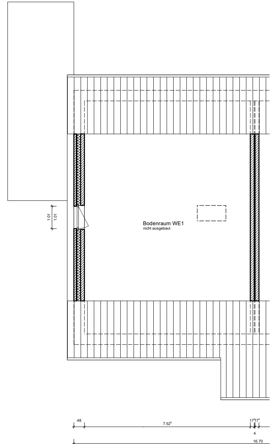
Dachgeschoss / Spitzboden
