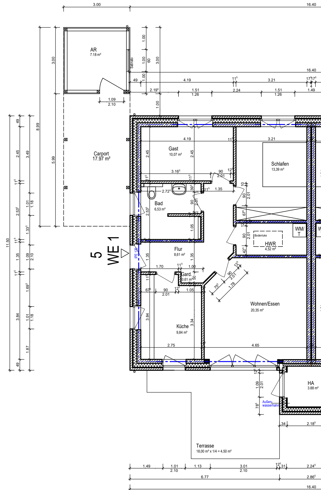
Erdgeschoss
