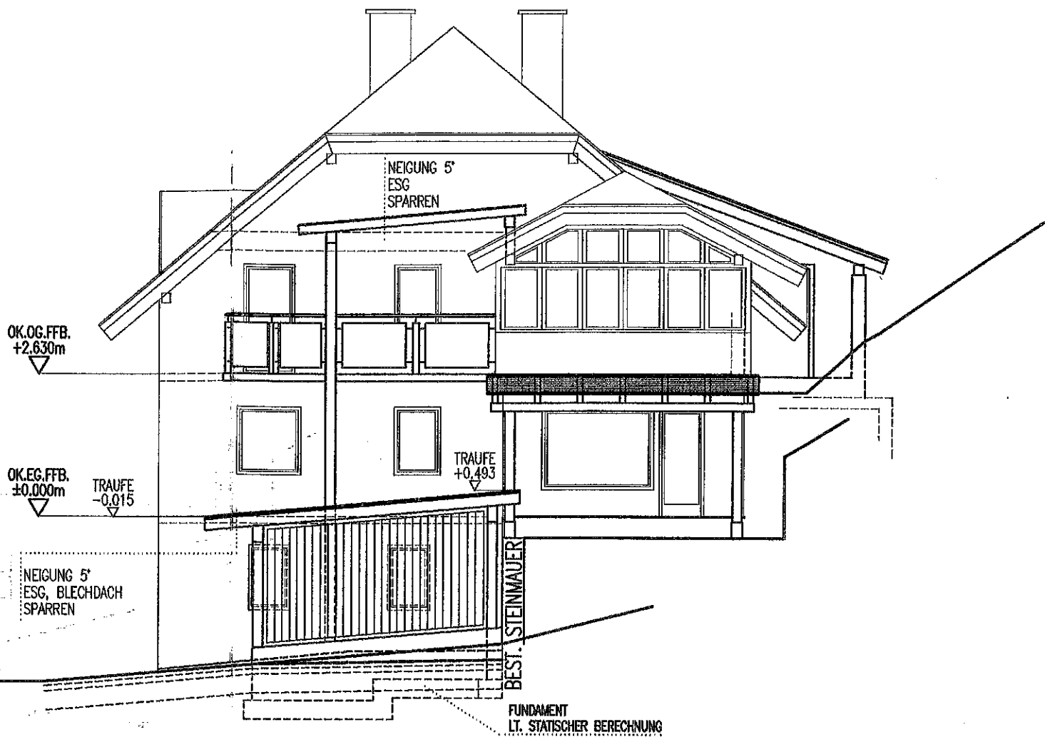
Ü D O S T A N S I C H T M 1:100
