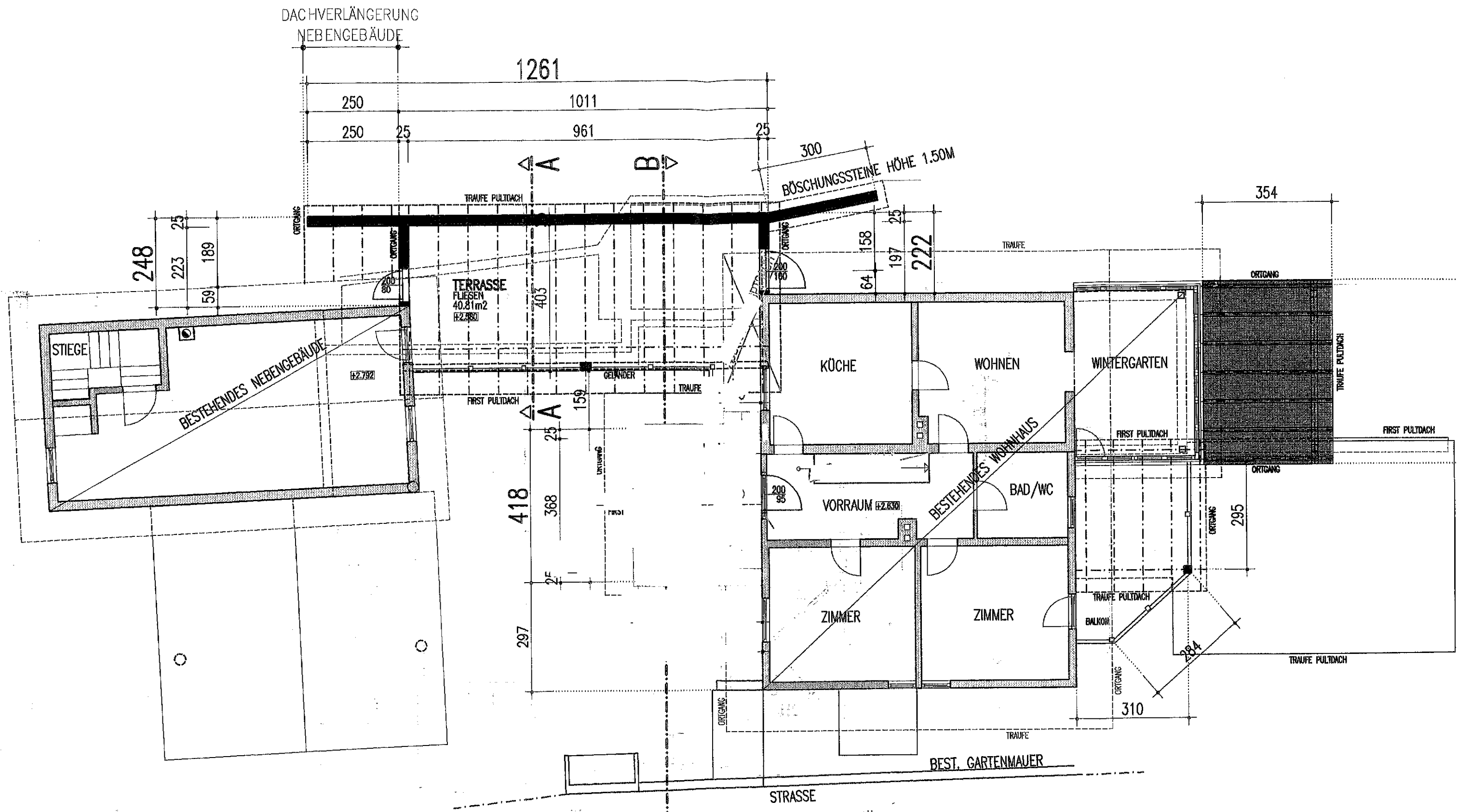
OBERGESCHOSS M 1:100
