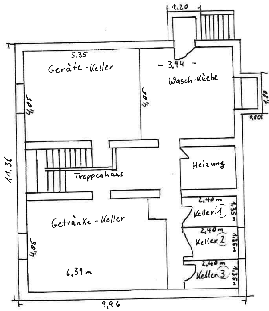
Kellergeschoß-Grundriß
