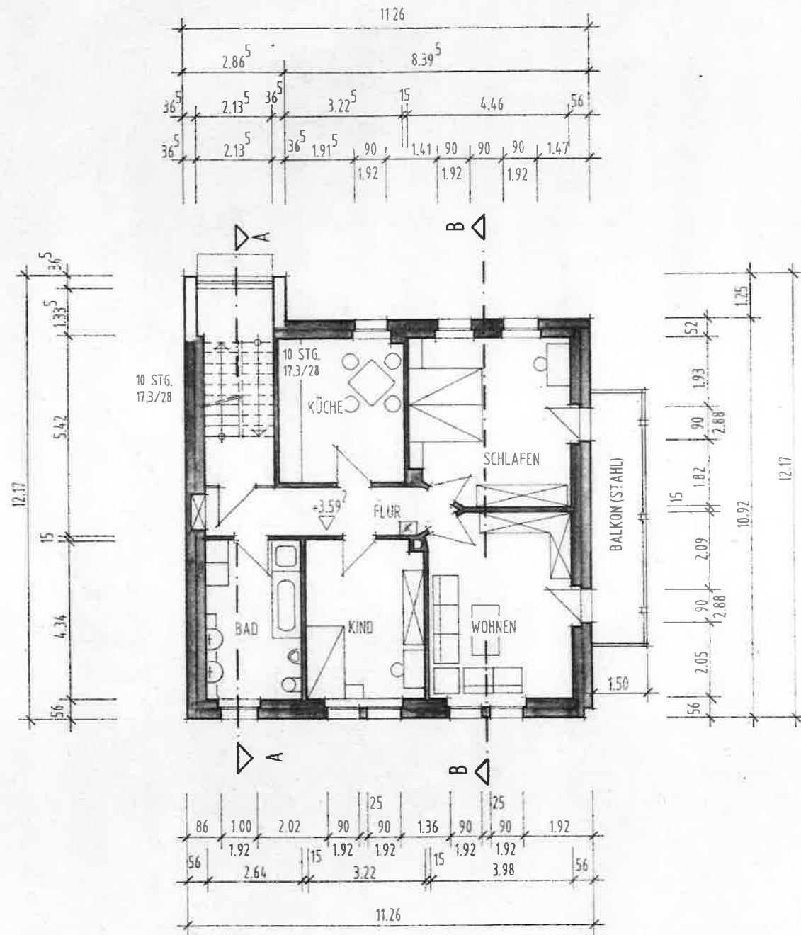
OBERGESCHOSS M. 1/100
