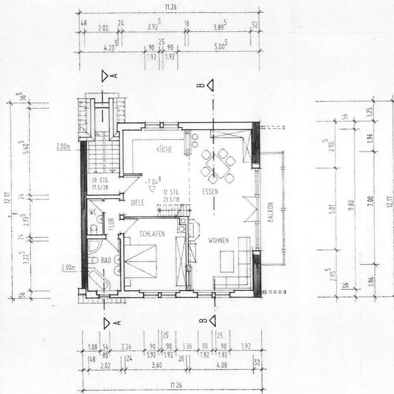
DACHGESCHOSS M. 1/100
