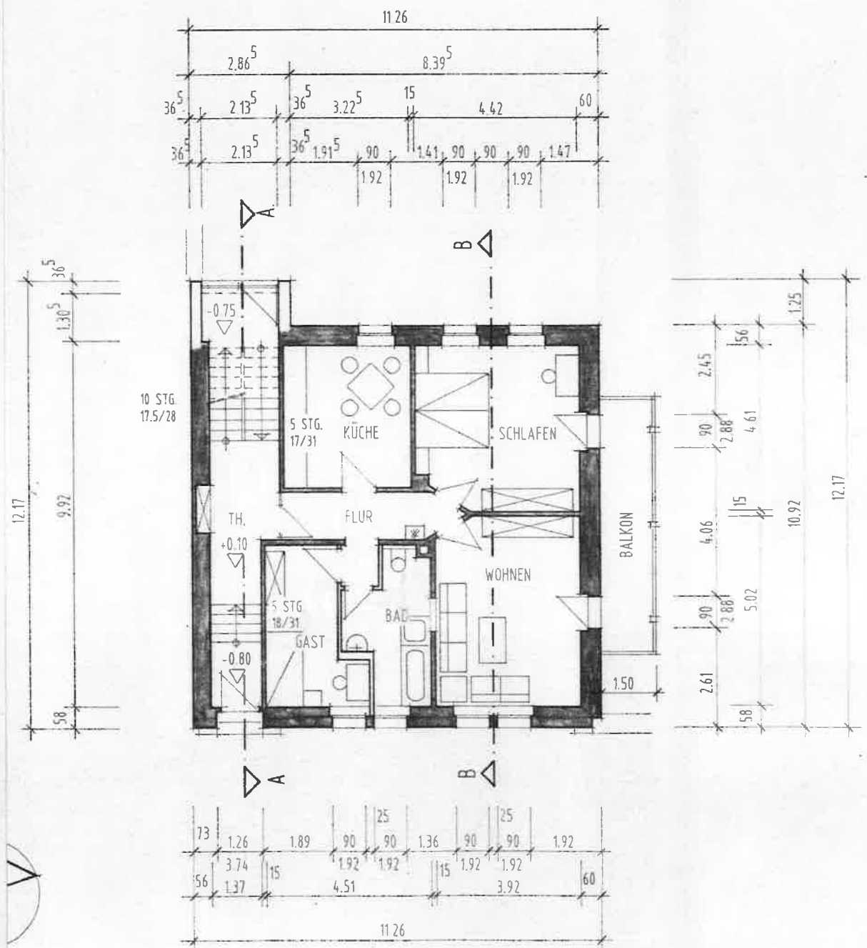
ERDGESCHOSS M. 1/100
