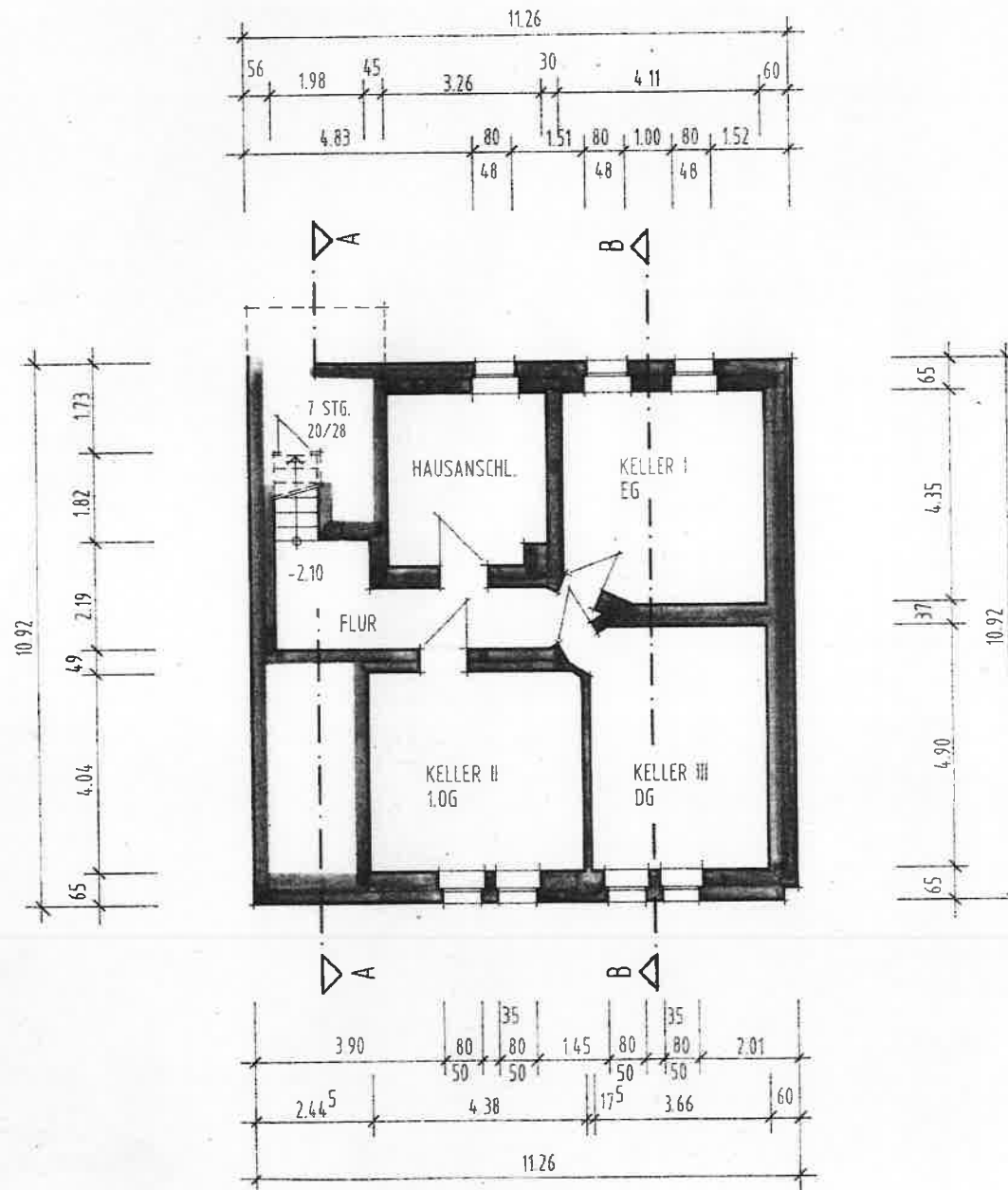
KELLERGEHOSS M. 1/100
