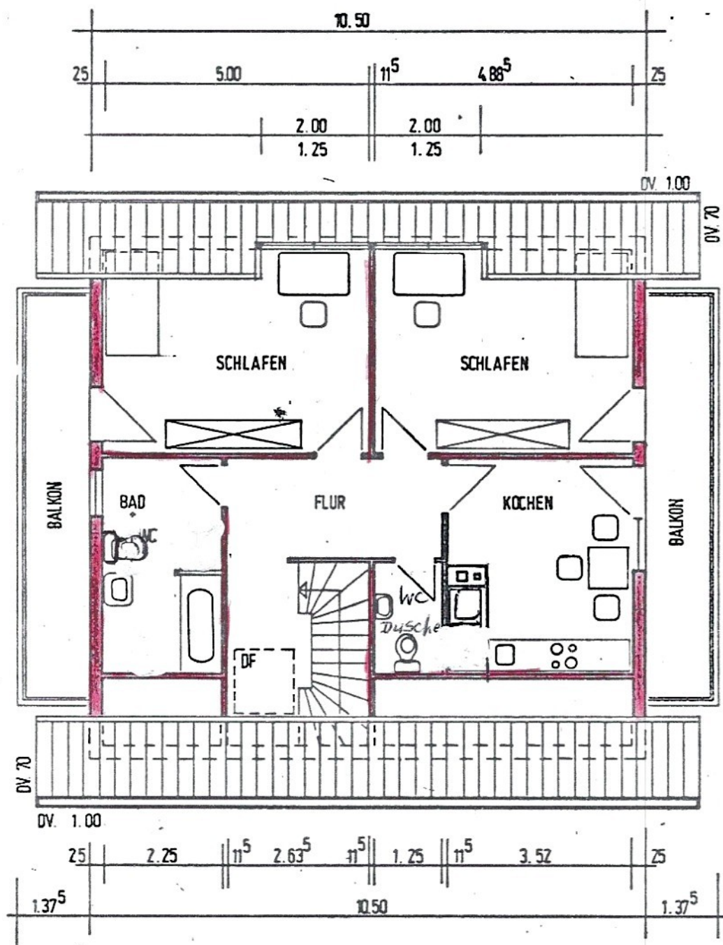
DACHGESCHOSS M. 1:100
