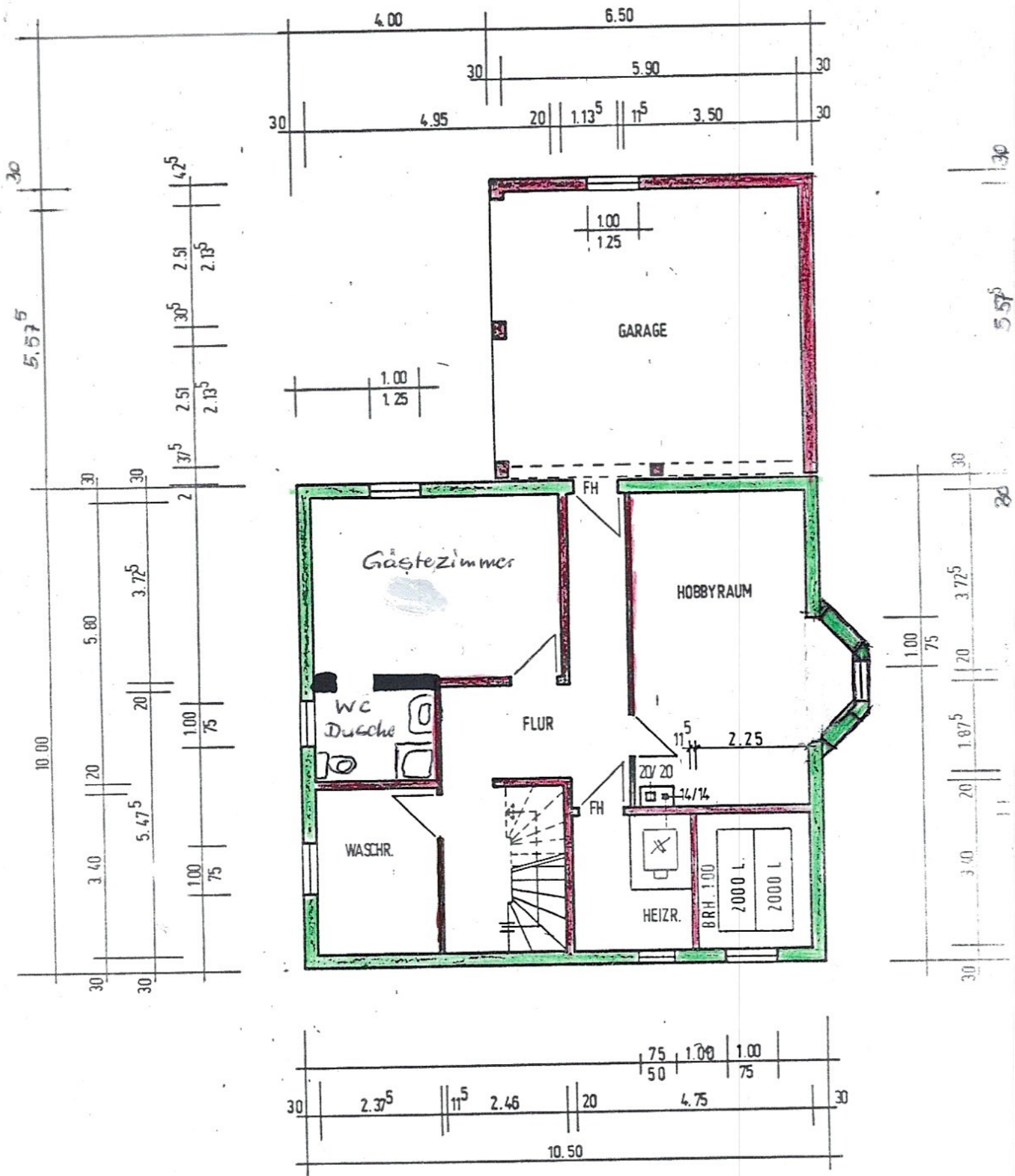
KELLERGECHOSS M. 1:100
