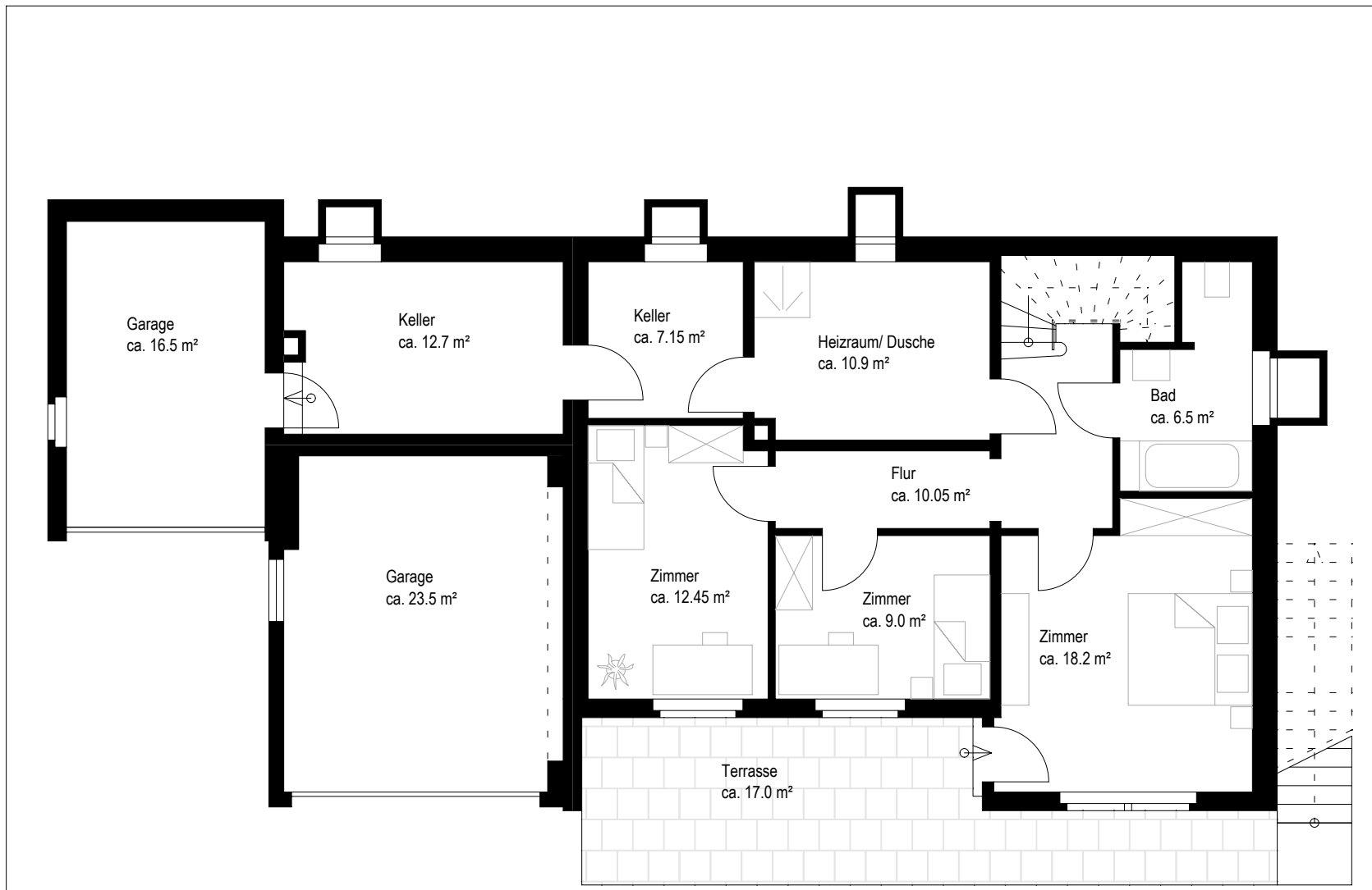
Grundriss Erdgeschoss ohne Maßstab
