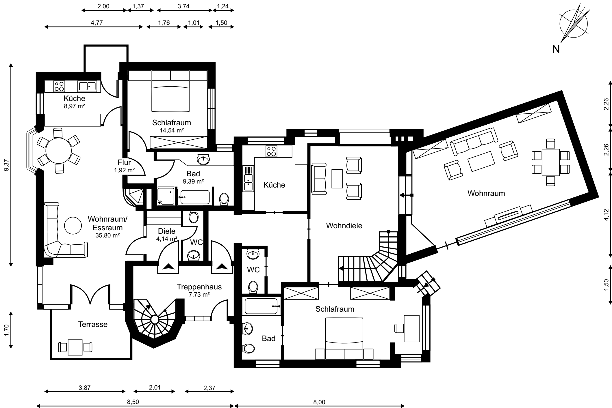
Erdgeschoss
