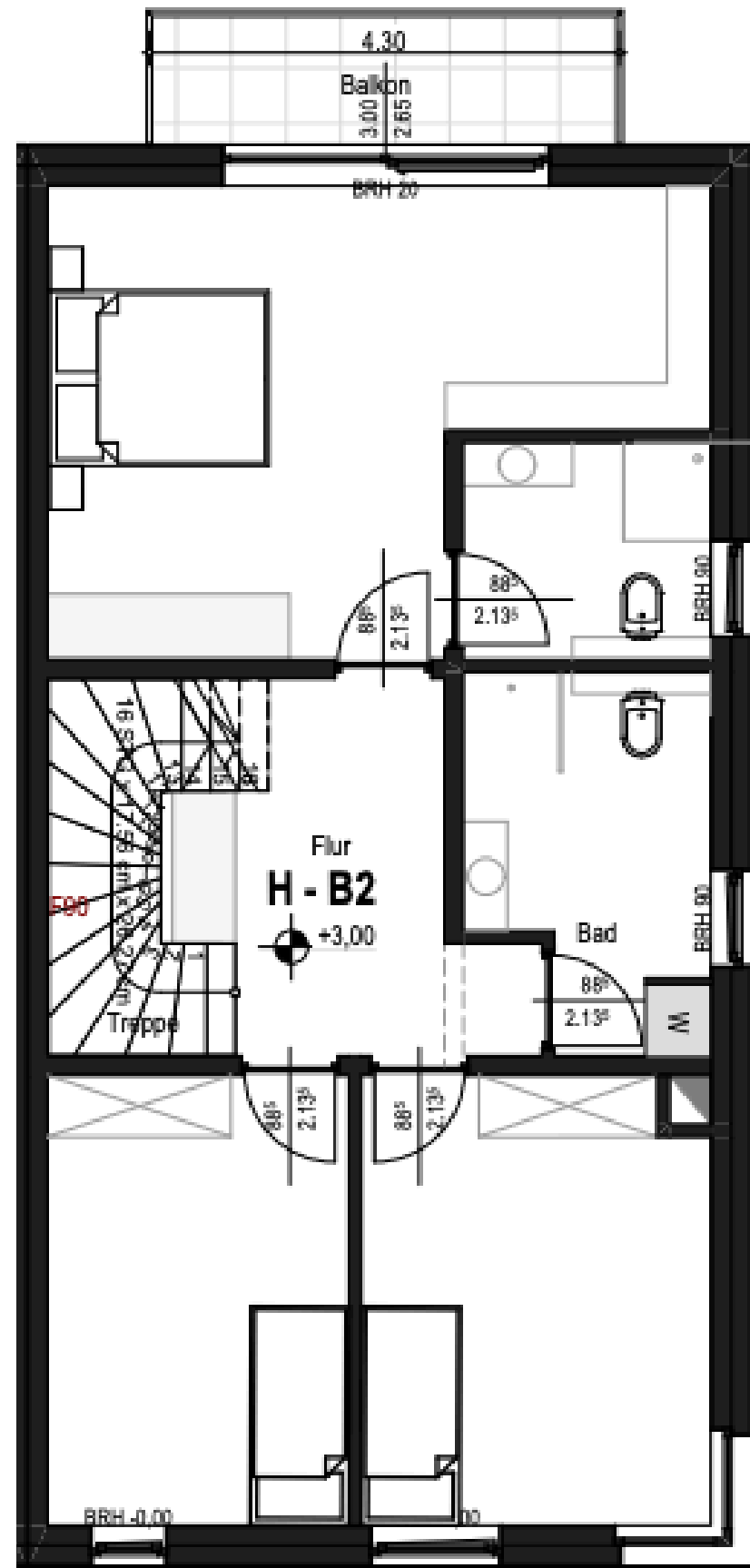
Grundriss Obergeschoss
