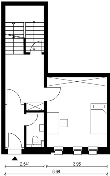
Erdgeschoss
