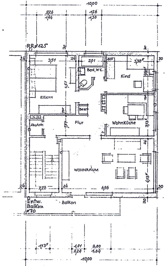
1. OBERGESCHOSS
