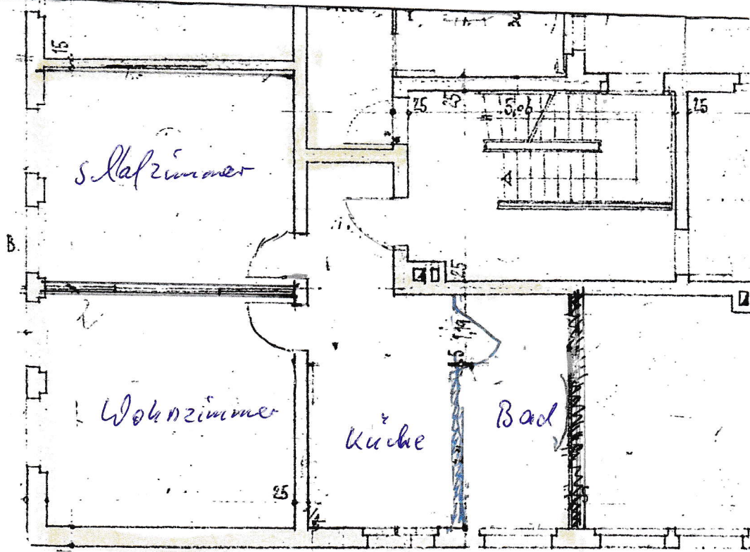
OBERGESCHOSS
