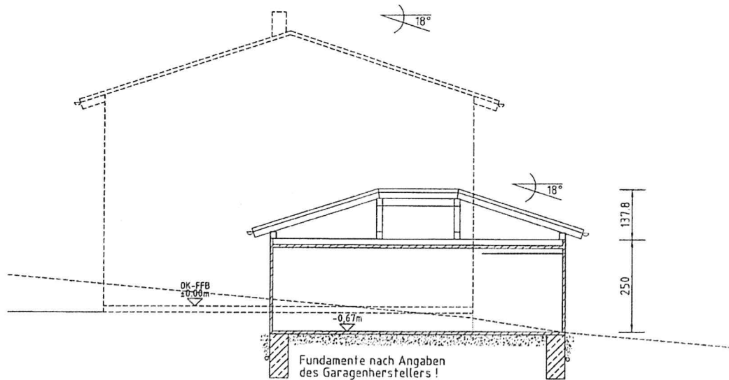
SCHNITT B-B
