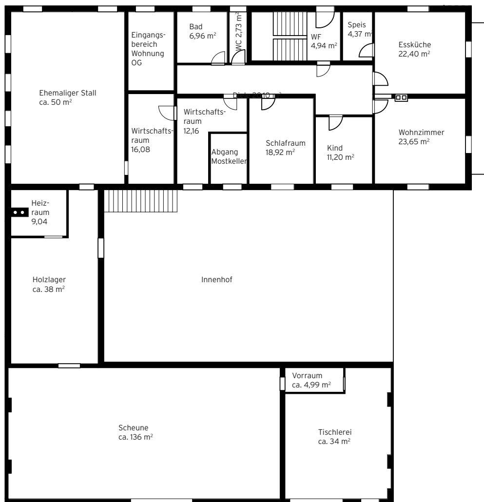
Grundrisse laut Plan, m 2 ohne Gewähr.
