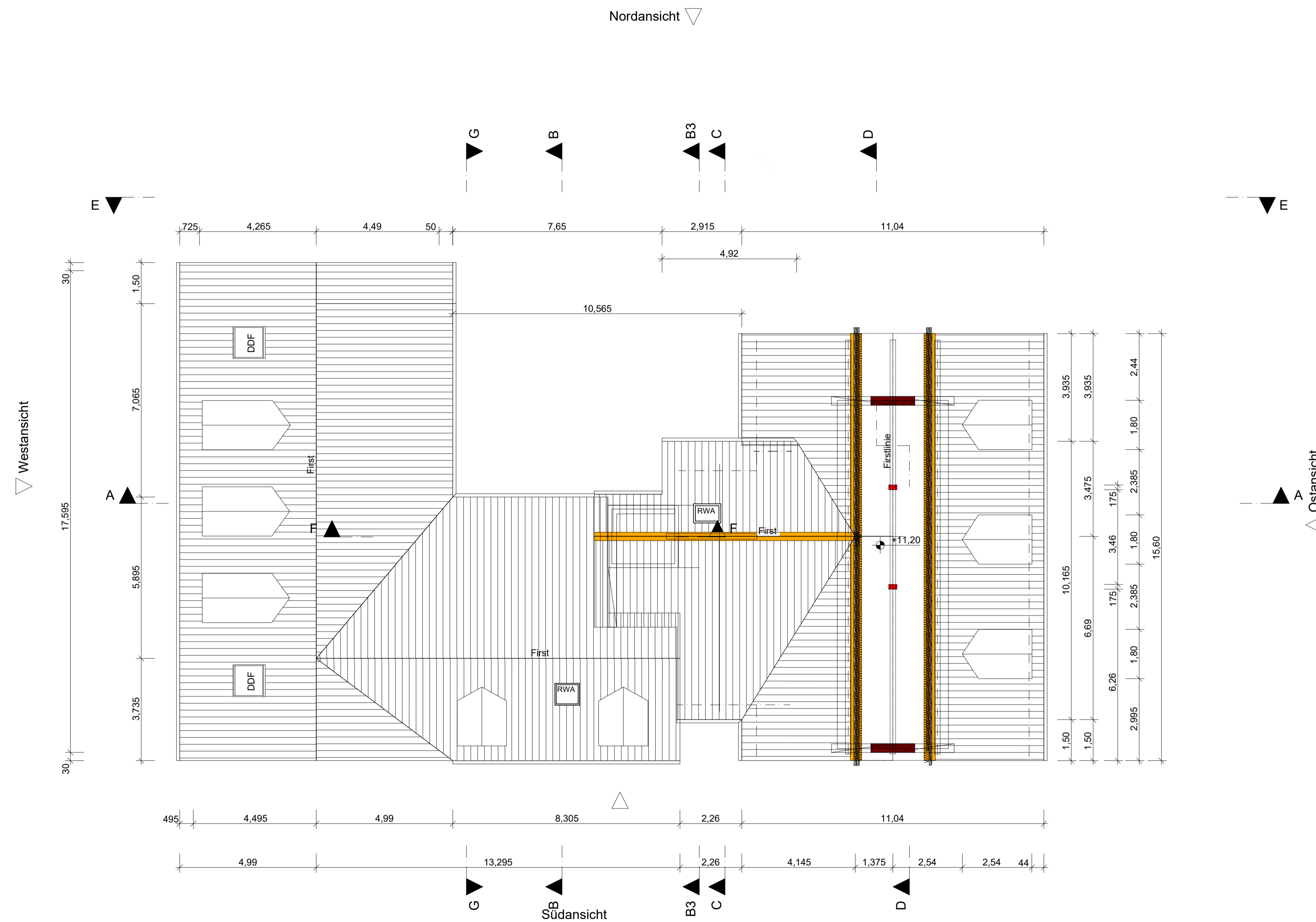
6. Dachaufsicht +11,30m 1:100
