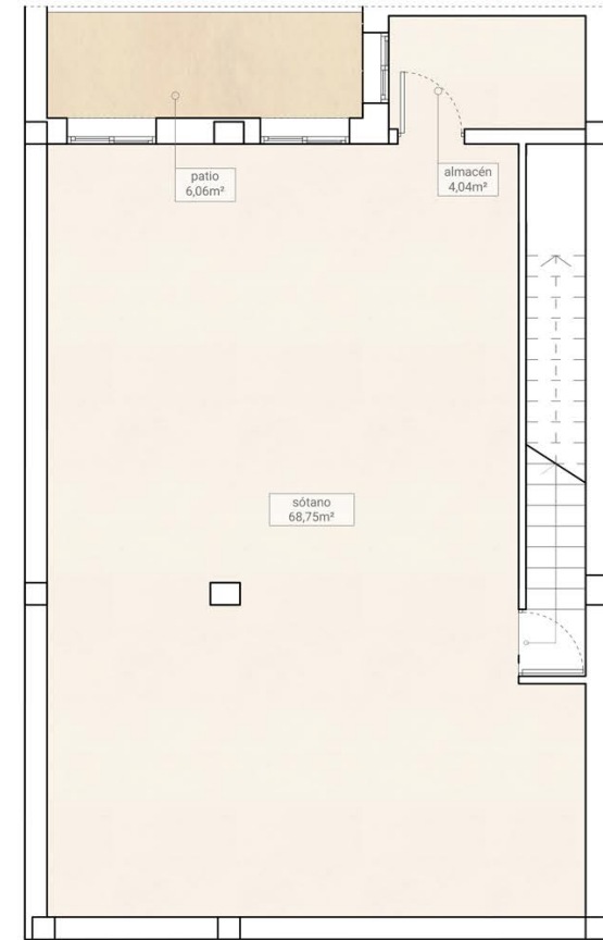
PLANTA SÓTANO/BASEMENT Superficies/Surfaces
