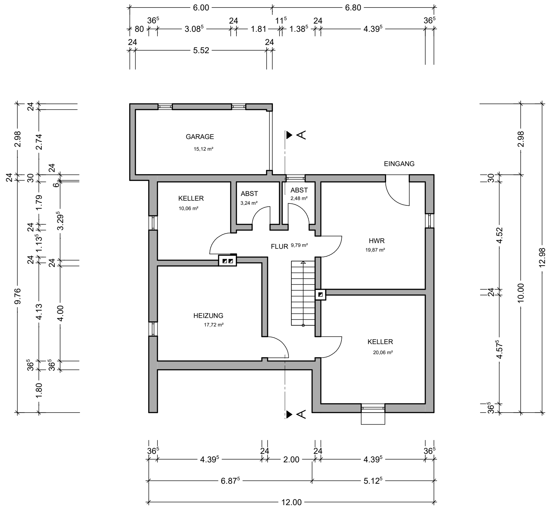
_kellergeschoss_
