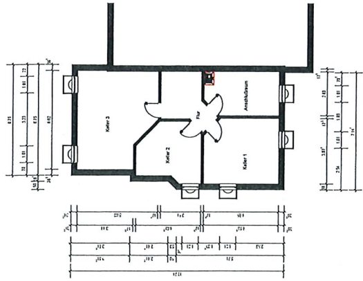
Kellergeschoss
