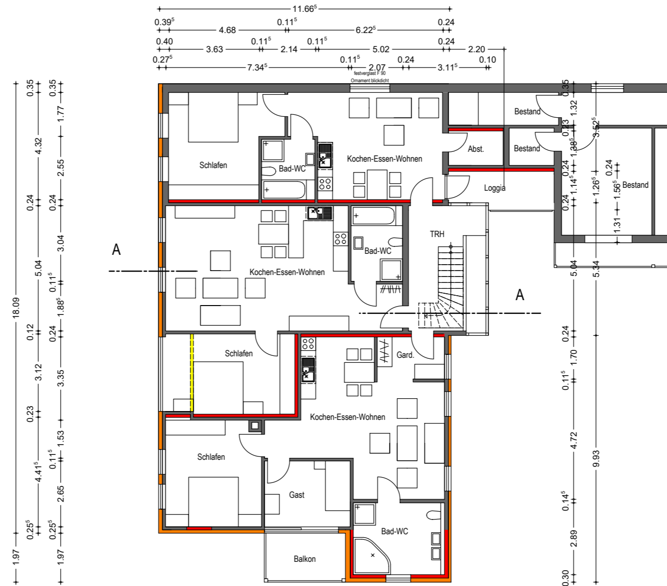
Obergeschossgrundriss
