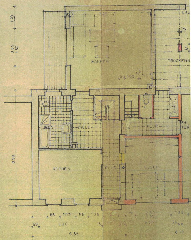
ERDGESCHOSS GRUNDRISS
