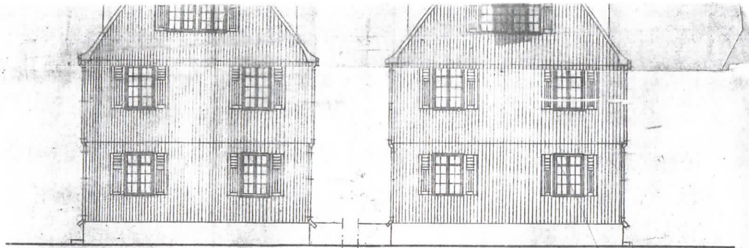
Ost-Ansicht
