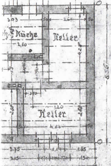
Kellergrundriss
