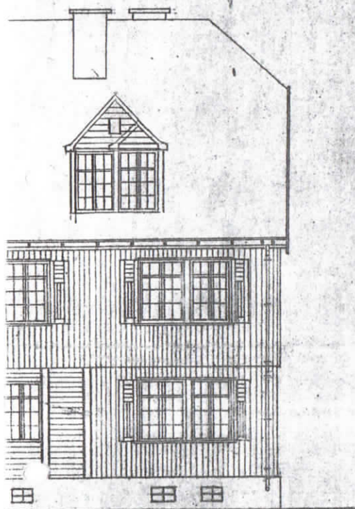
Strassenansicht.
