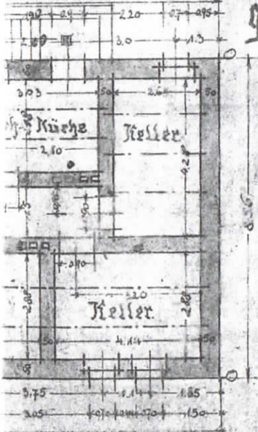
Kellergrundriss
