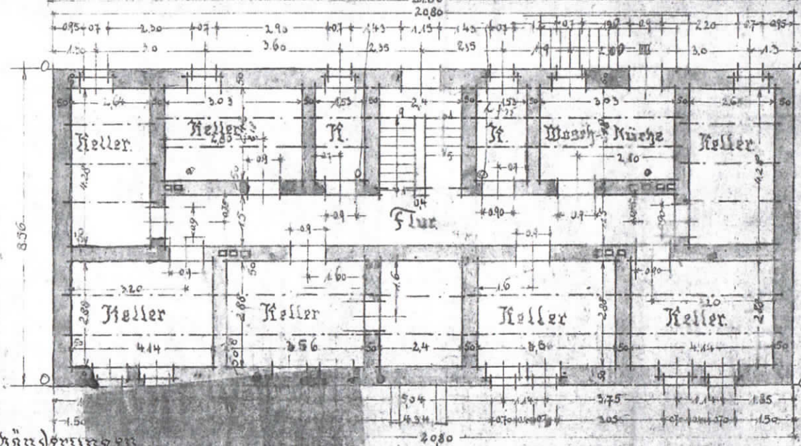
Übergeschoss- grundriss.
