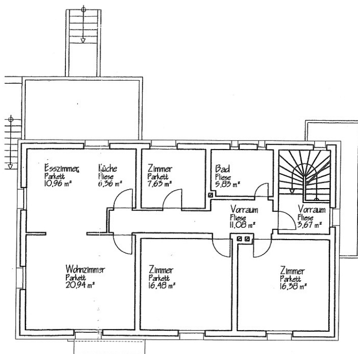
2. OBERGESCHOSS BESTAND
