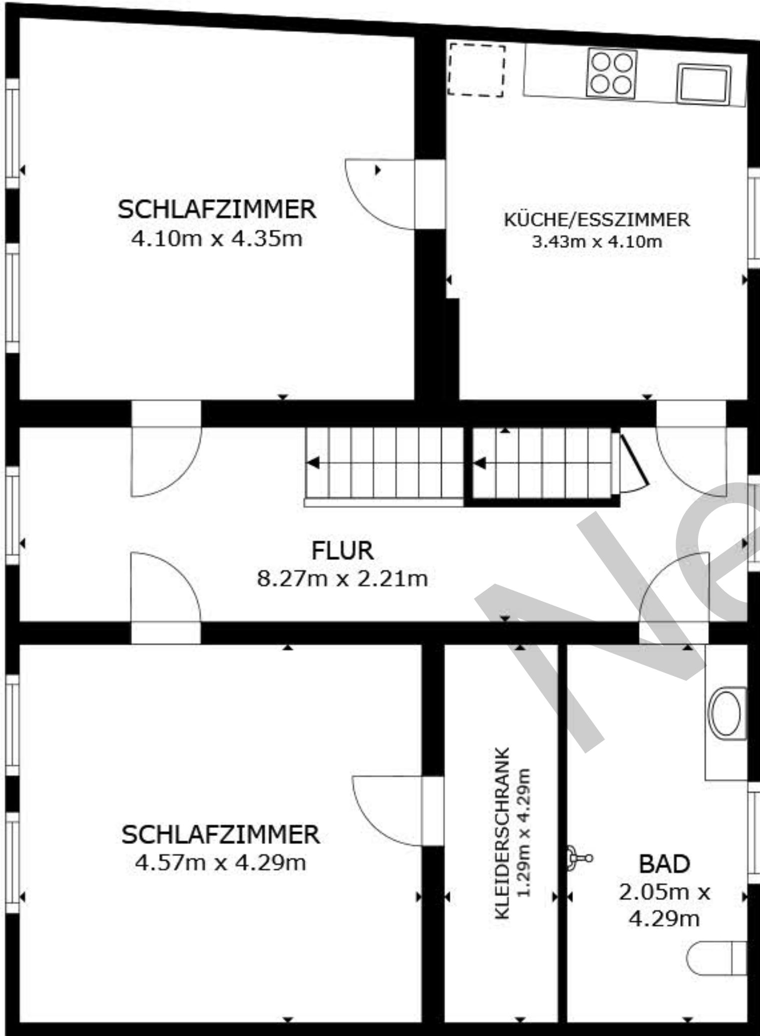
Obergeschoss
