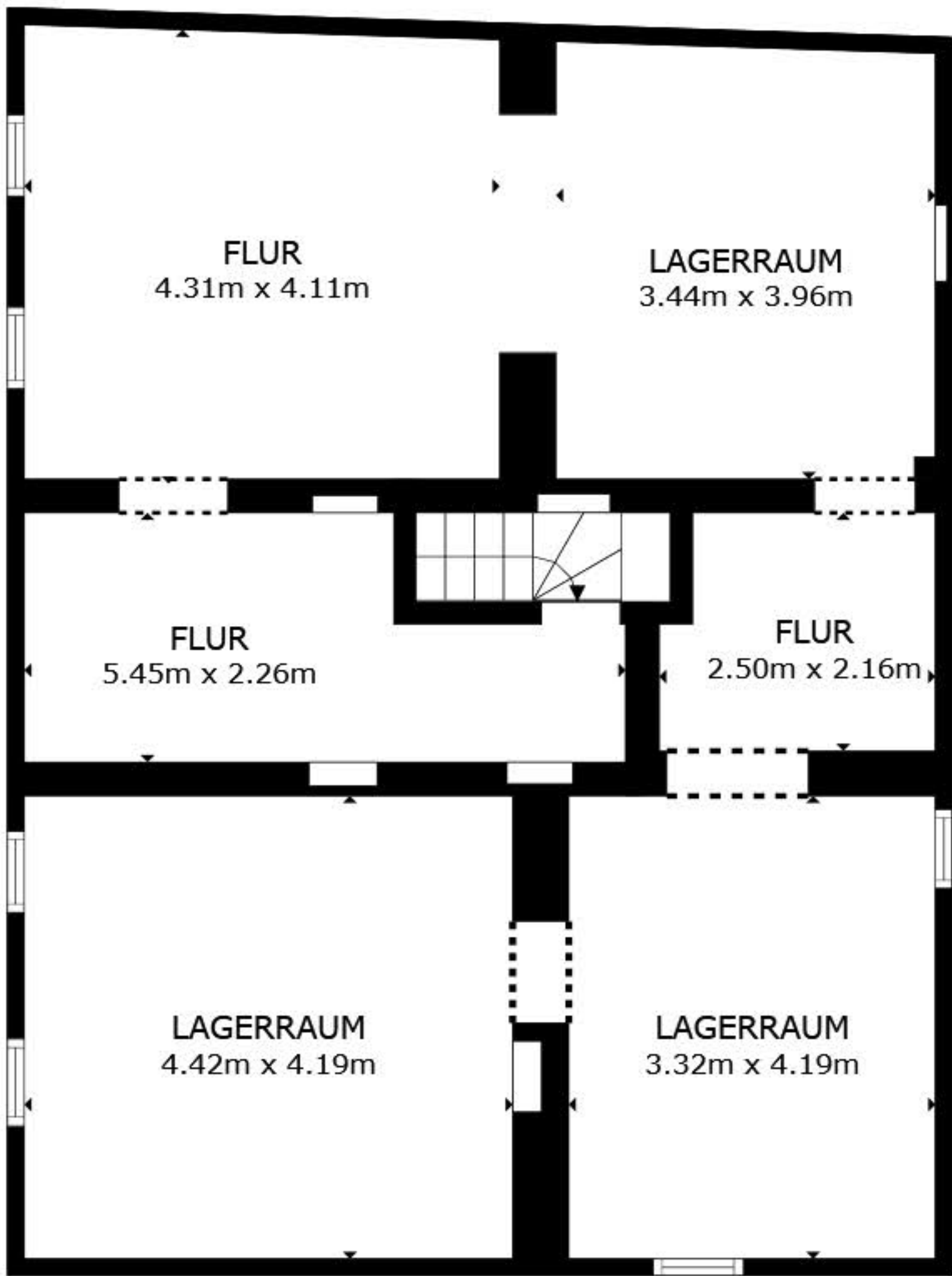
Keller
