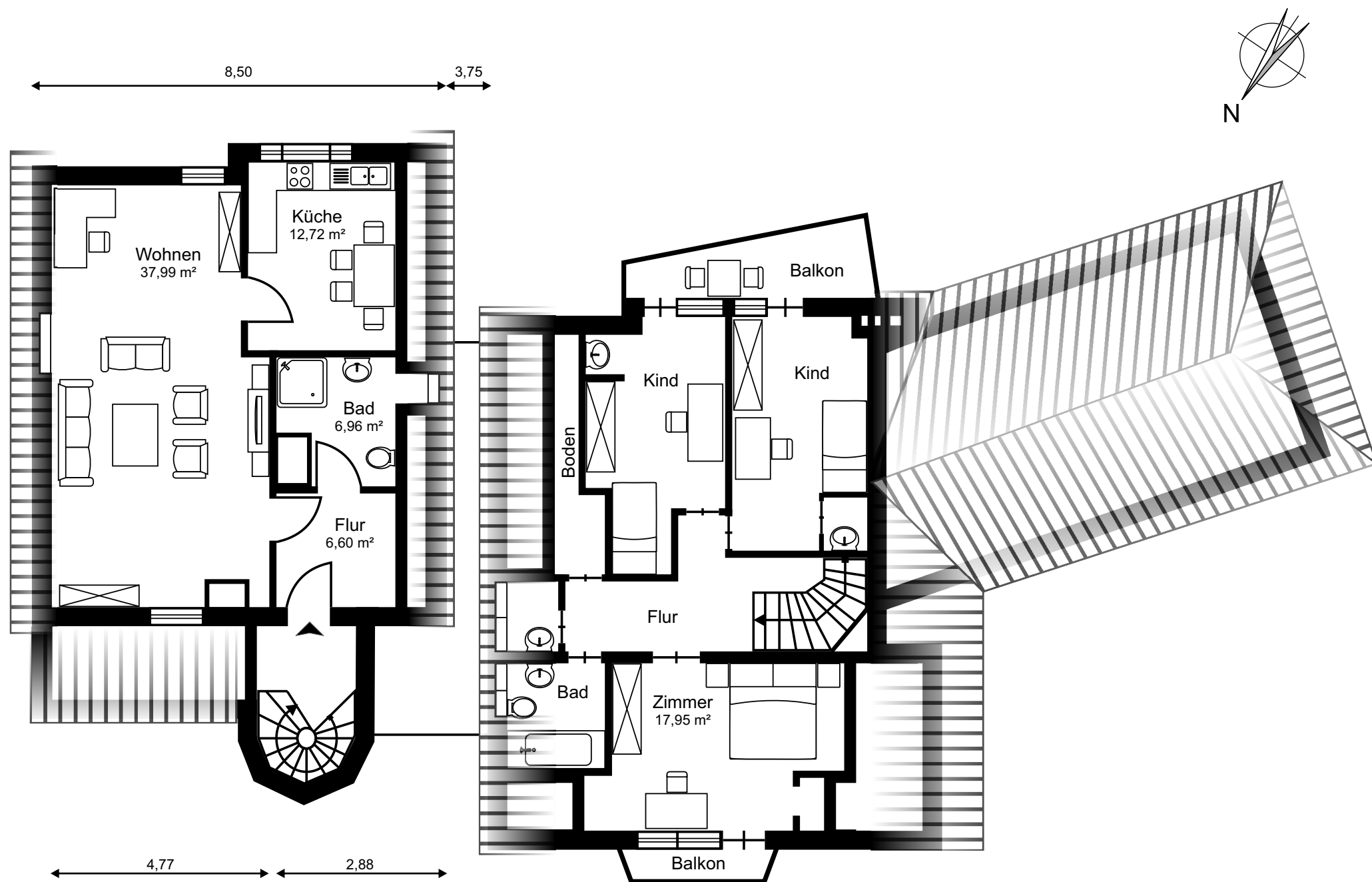
Obergeschoss
