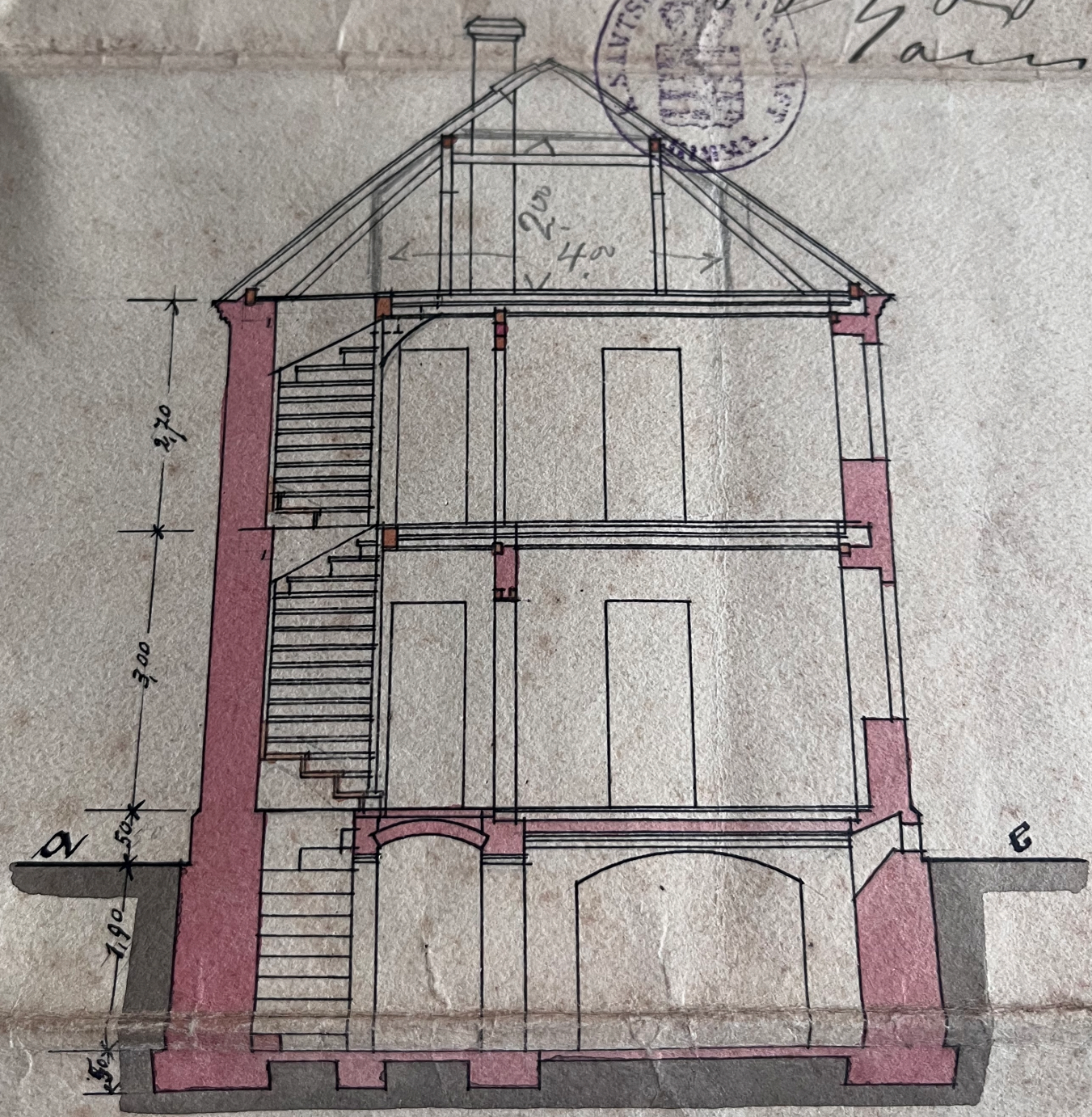
Schnitt.
