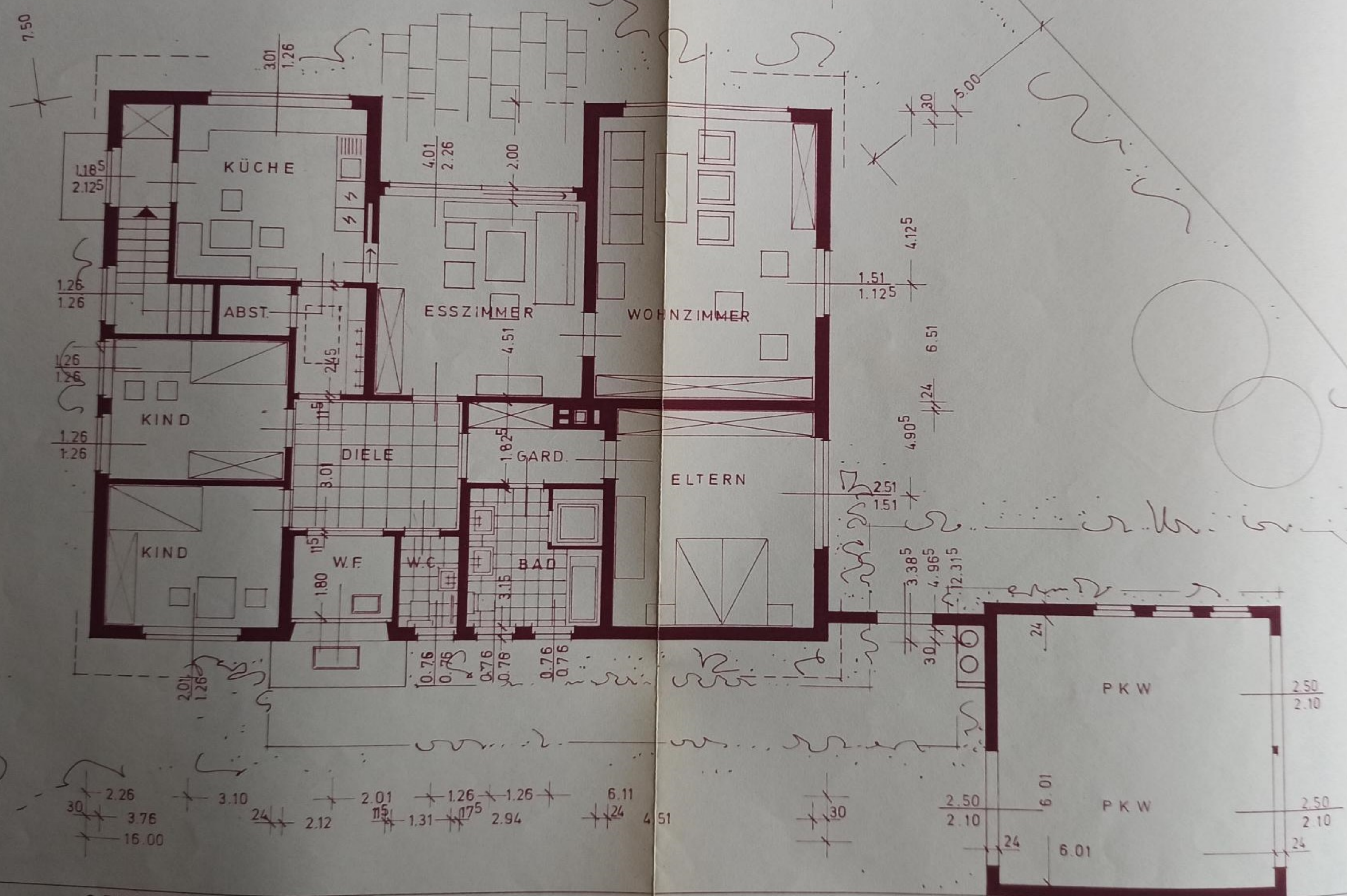
GRUNDRISS ERDGESCHOSS
