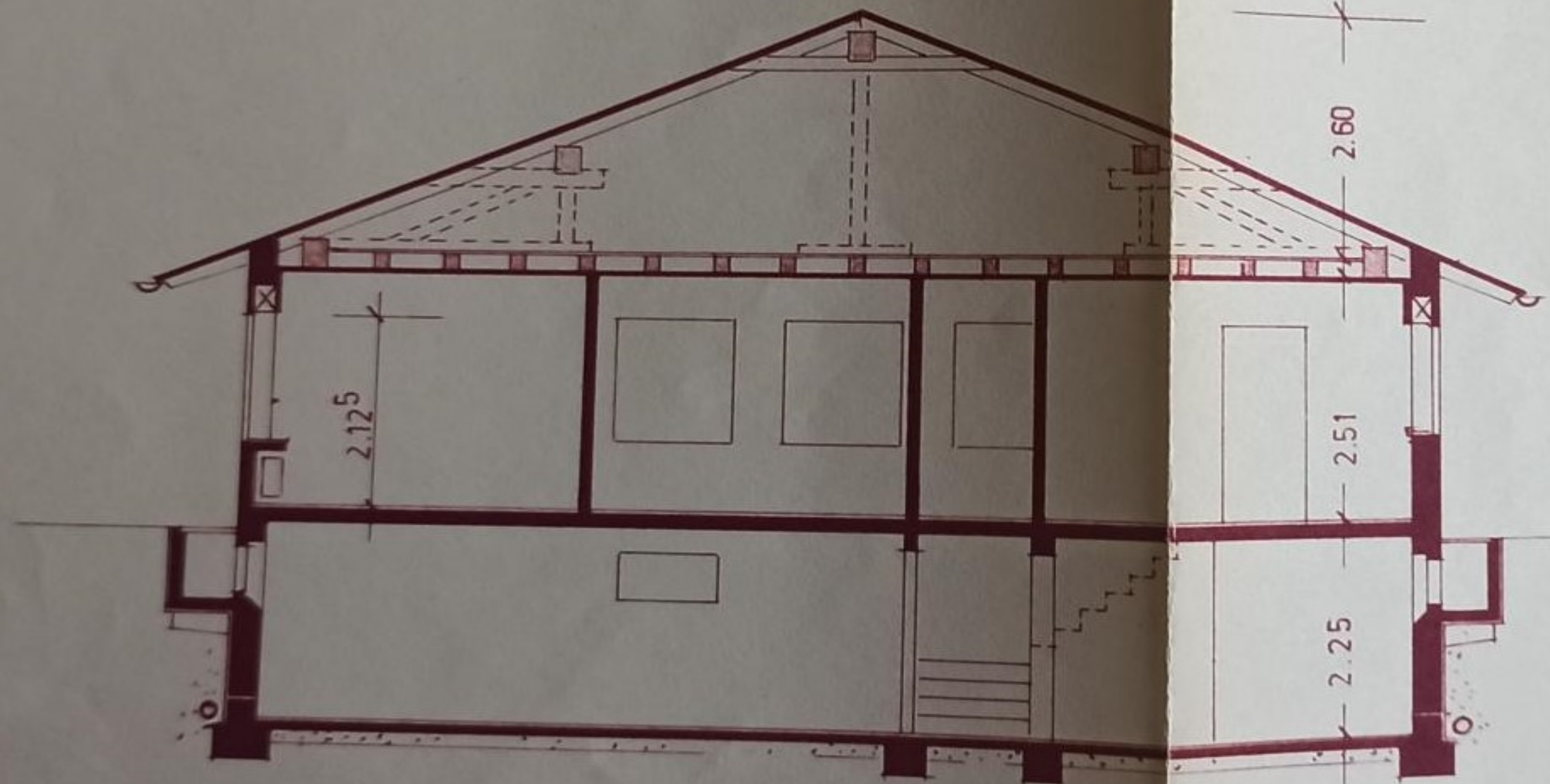
SCHNITT WOHNHAUS
