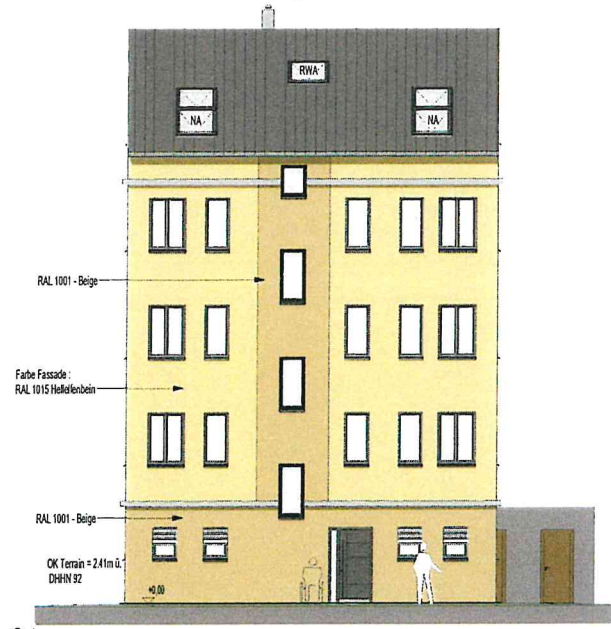
Ost M 1 : 100
