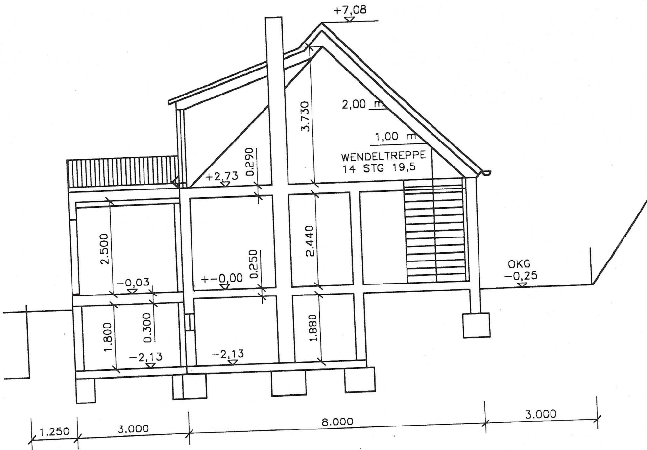
SCHNITT
