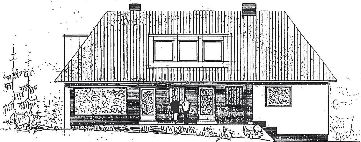
Ansicht von Osten M 1:100
