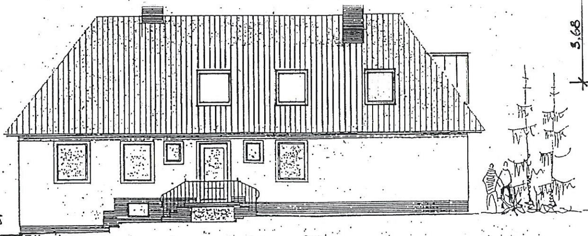
Ansicht von Westen M 1:100
