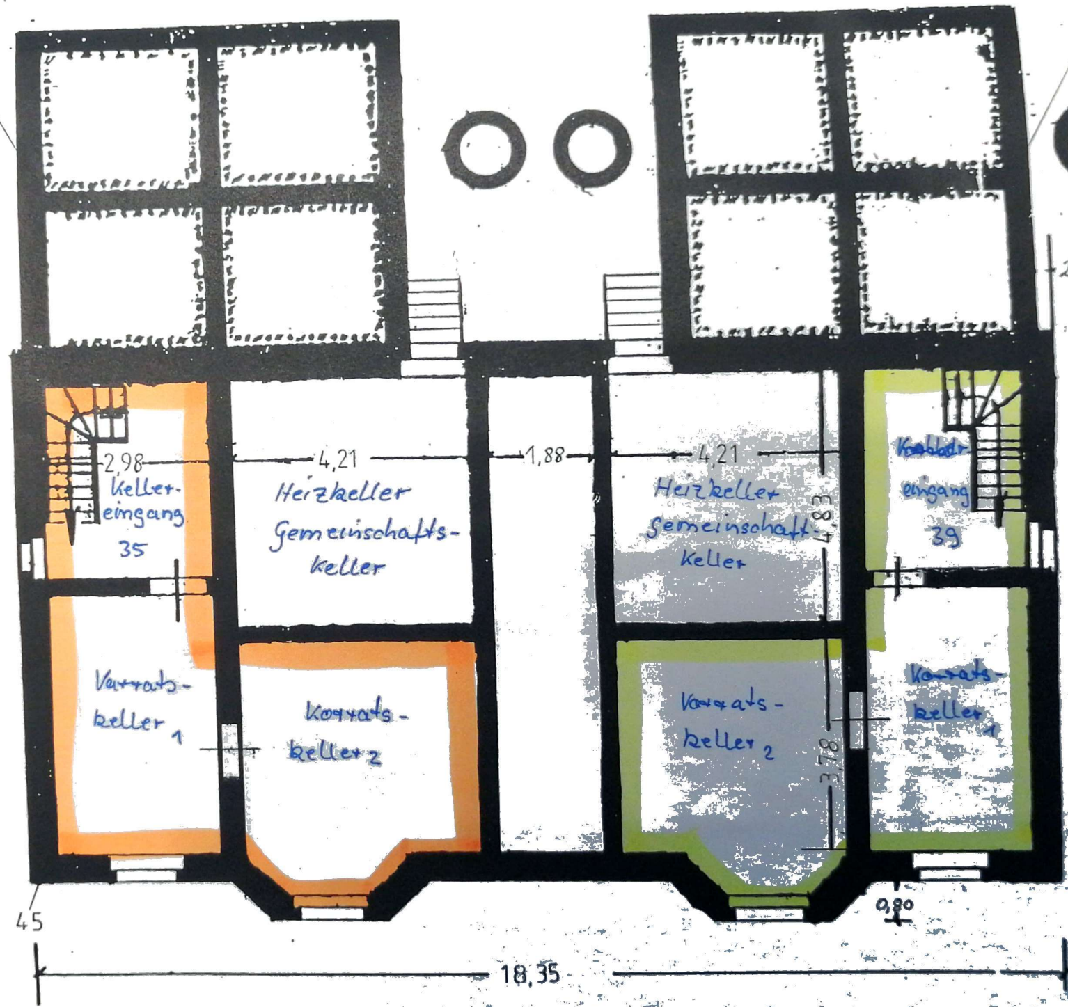
Kellergeschoss
