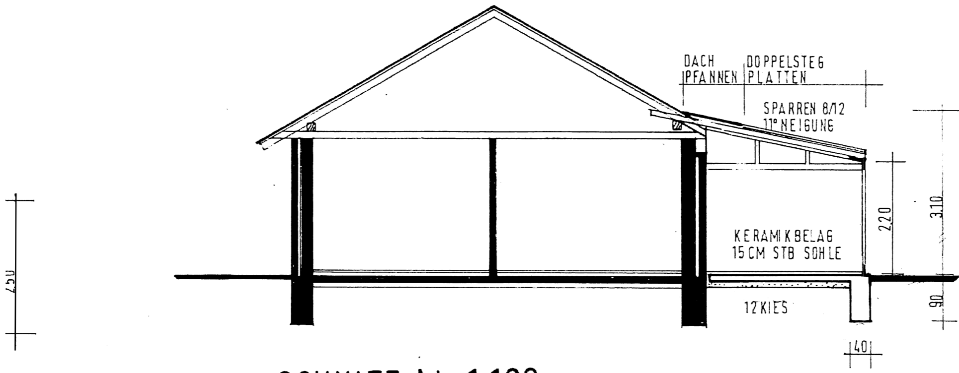
SCHNITT M-1:100
