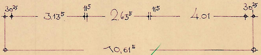
GRUNDRISS • DACHGESCHOSS
