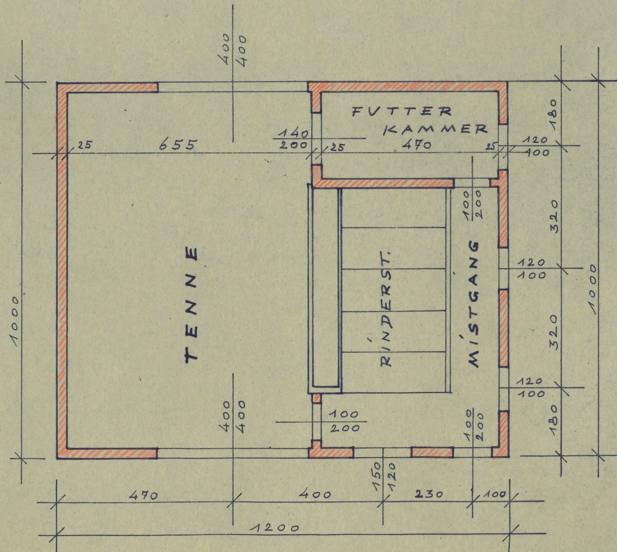
ERDGESCHOSSGRUNDRISS
