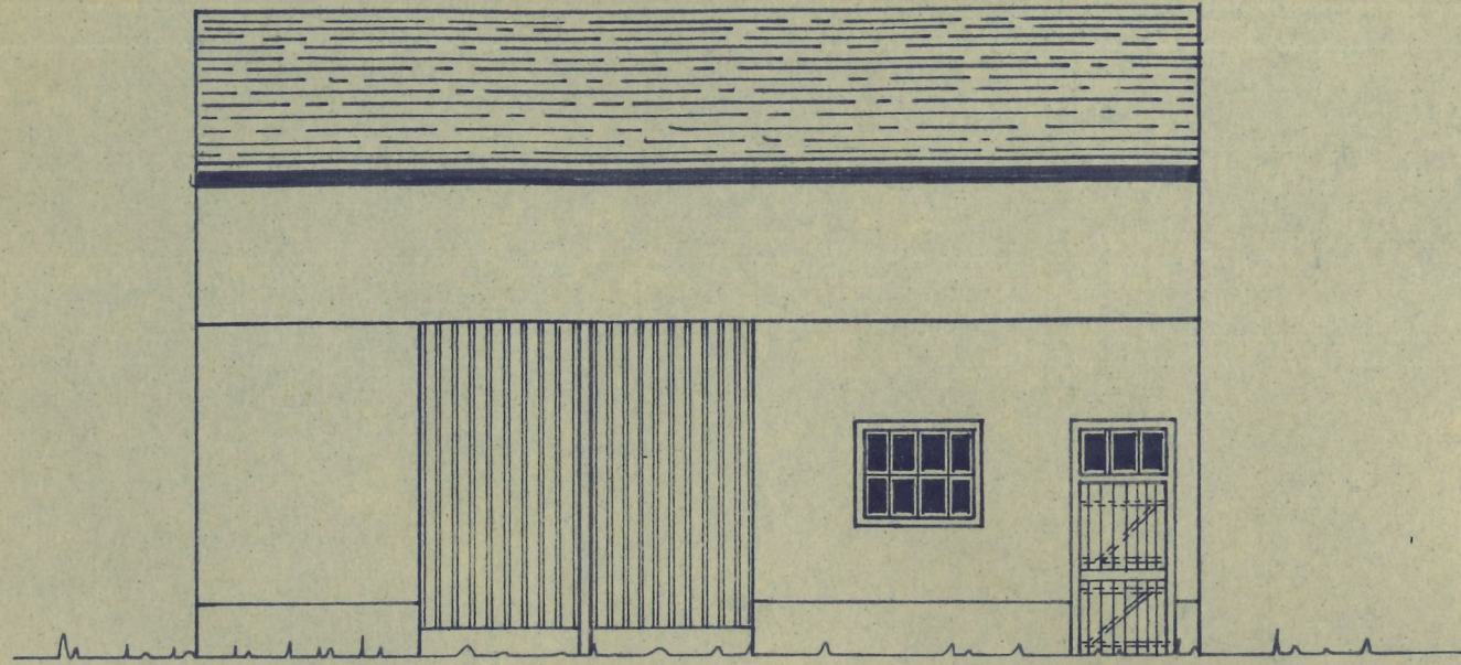
HOFANSICHT
