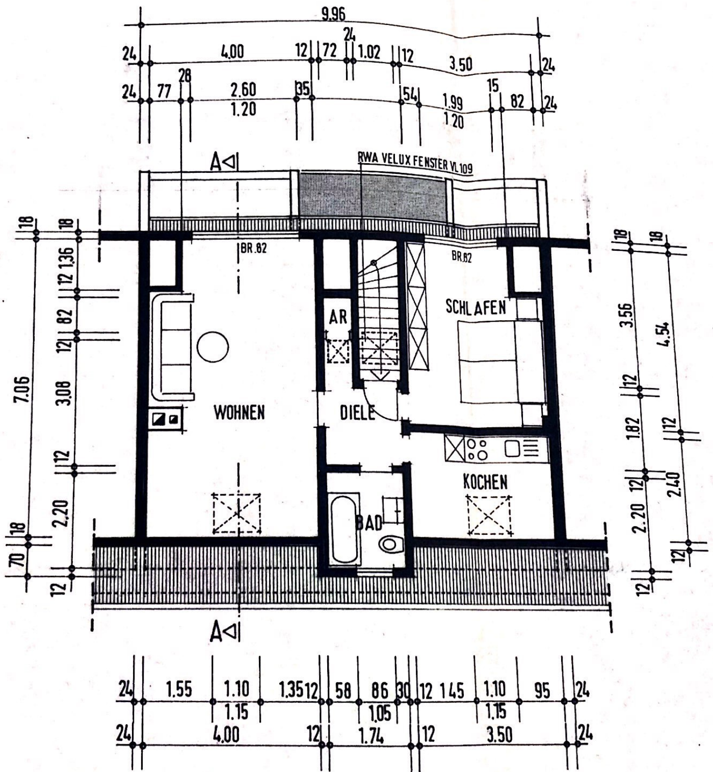
DACHGESCHOSS GRUNDRISS
