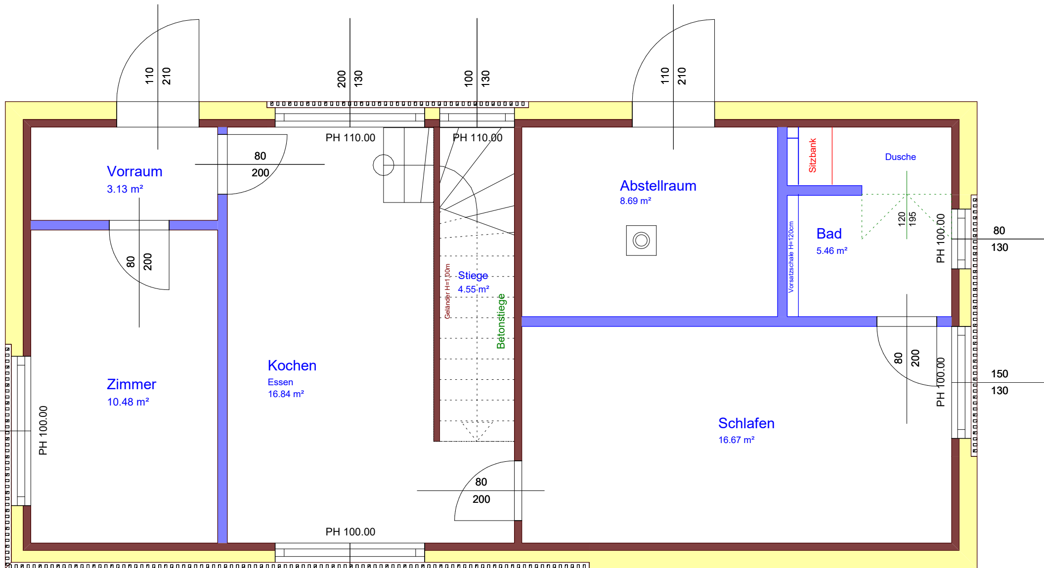
VARIANTE 1 OBERGESCHOSS
