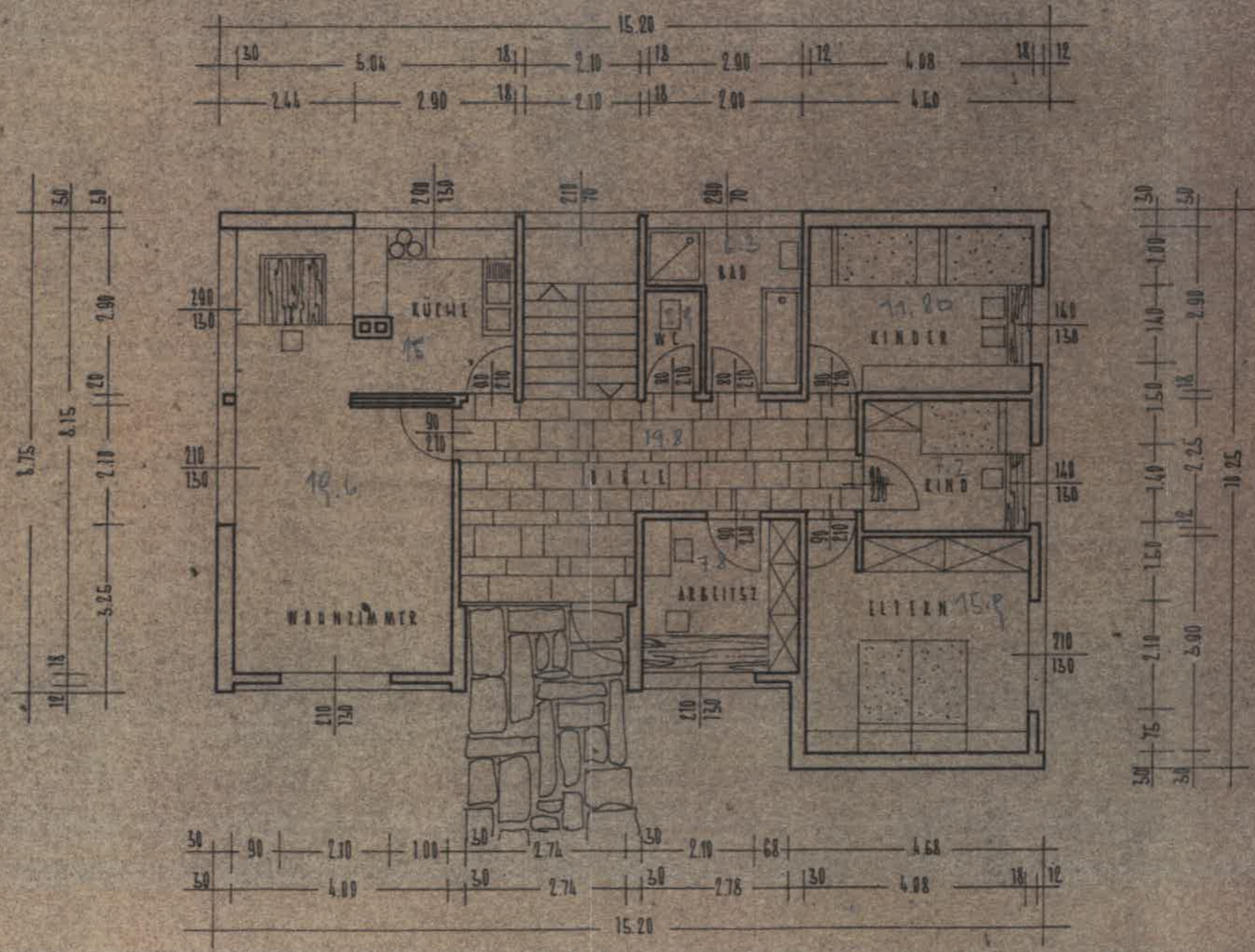
ERDGESCHOSS M: 1:100
