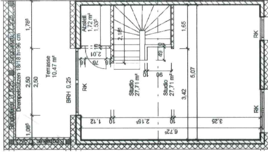
Grundriss 2. Obergeschoss
