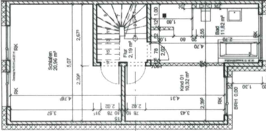
Grundriss 1. Obergeschoss
