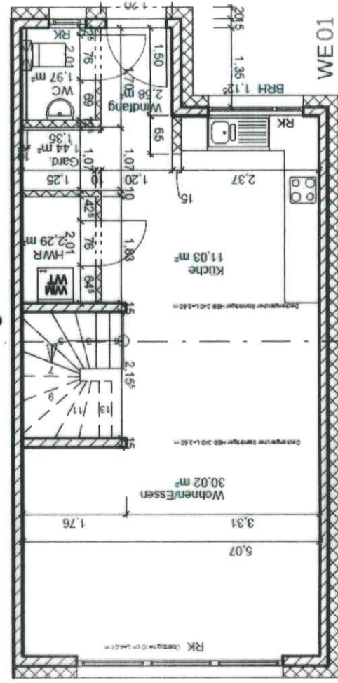
Grundriss Erdgeschoss
