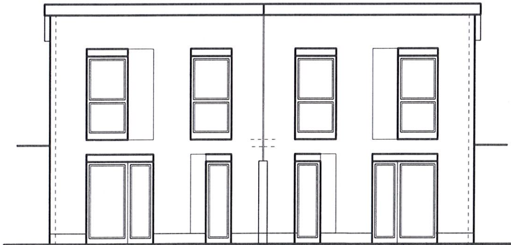
TERRASSENANSICHT
