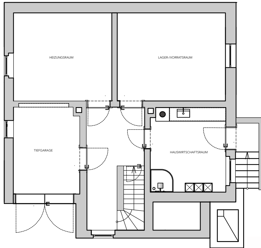
KELLERGESCHOSS (ohne Maßstab)
