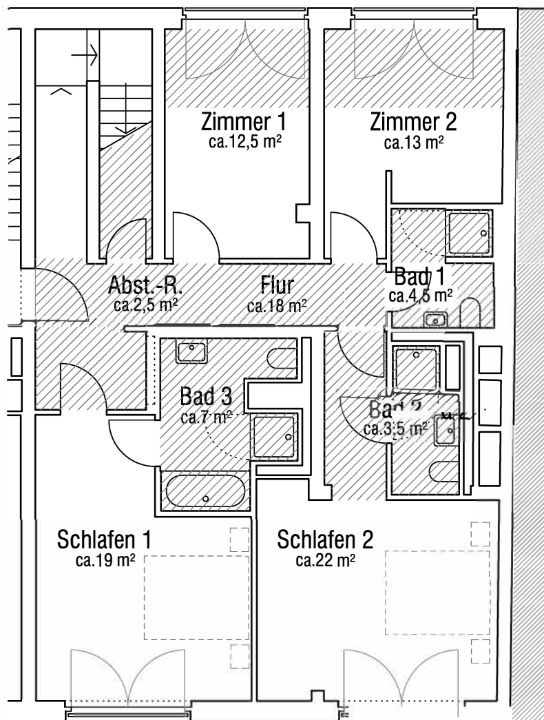
Wohnung 26 (unten) im VI. Obergeschoss
