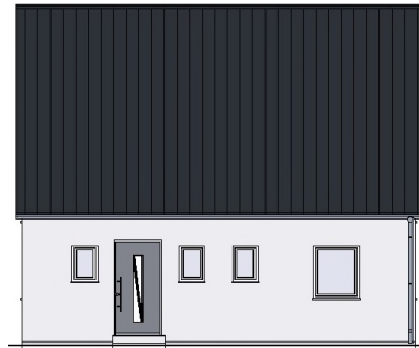
Eingang Nordansicht
