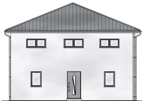
Eingang Nordansicht
