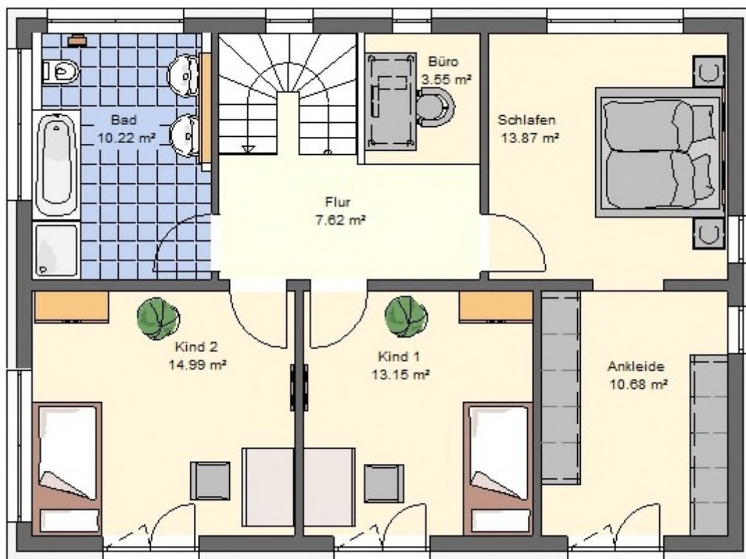
Obergeschoss
