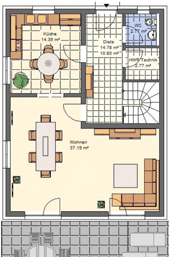
(Terrasse) Erdgeschoss
