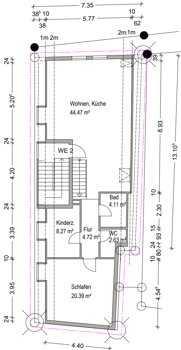
Grundriss DG
