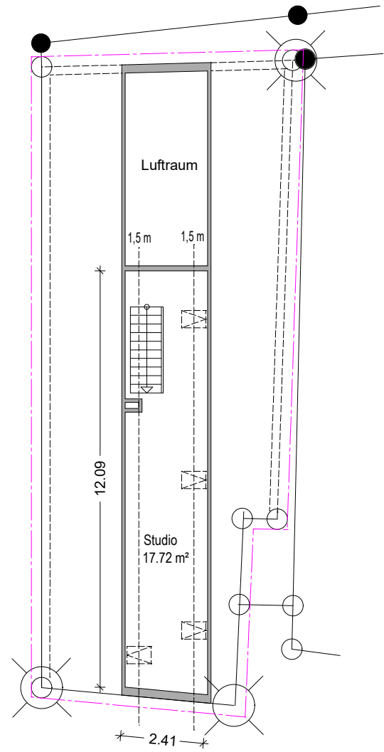
Grundriss Spitzboden
