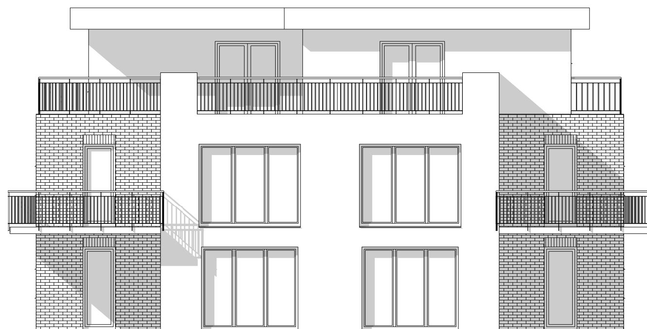
SÜD - ANSICHT
