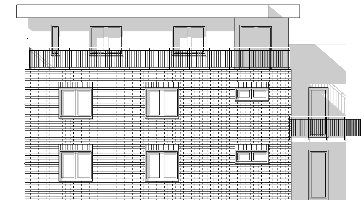
WEST - ANSICHT
