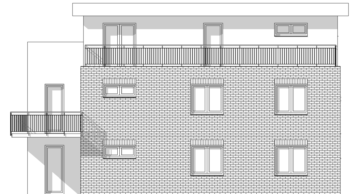
OST - ANSICHT
