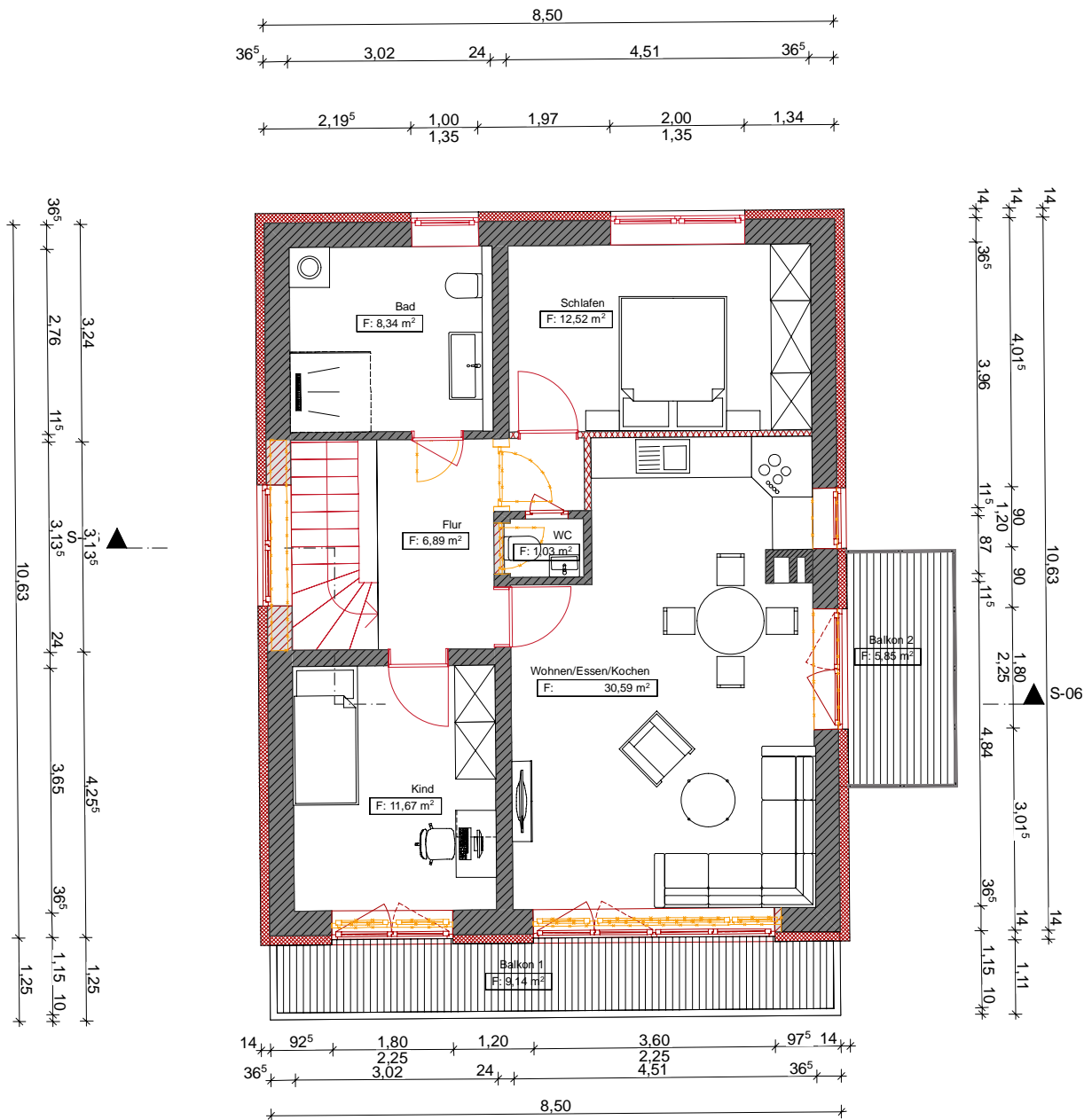
Obergeschoss Nachbar Am Strasserfeld 1:100
