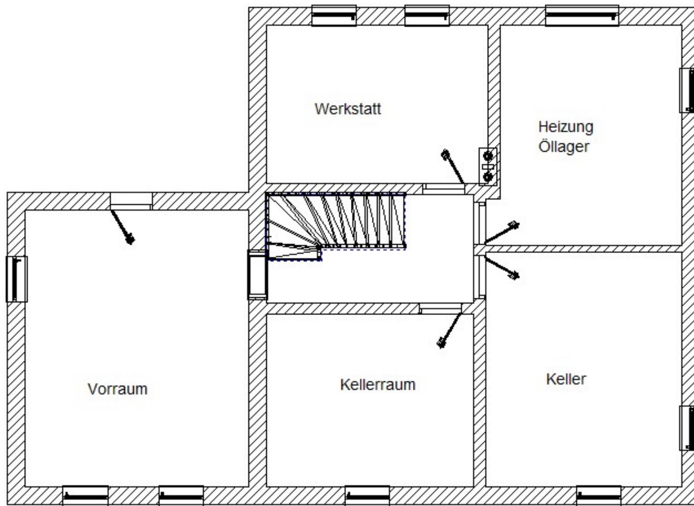
Skizze Kellergeschoss
