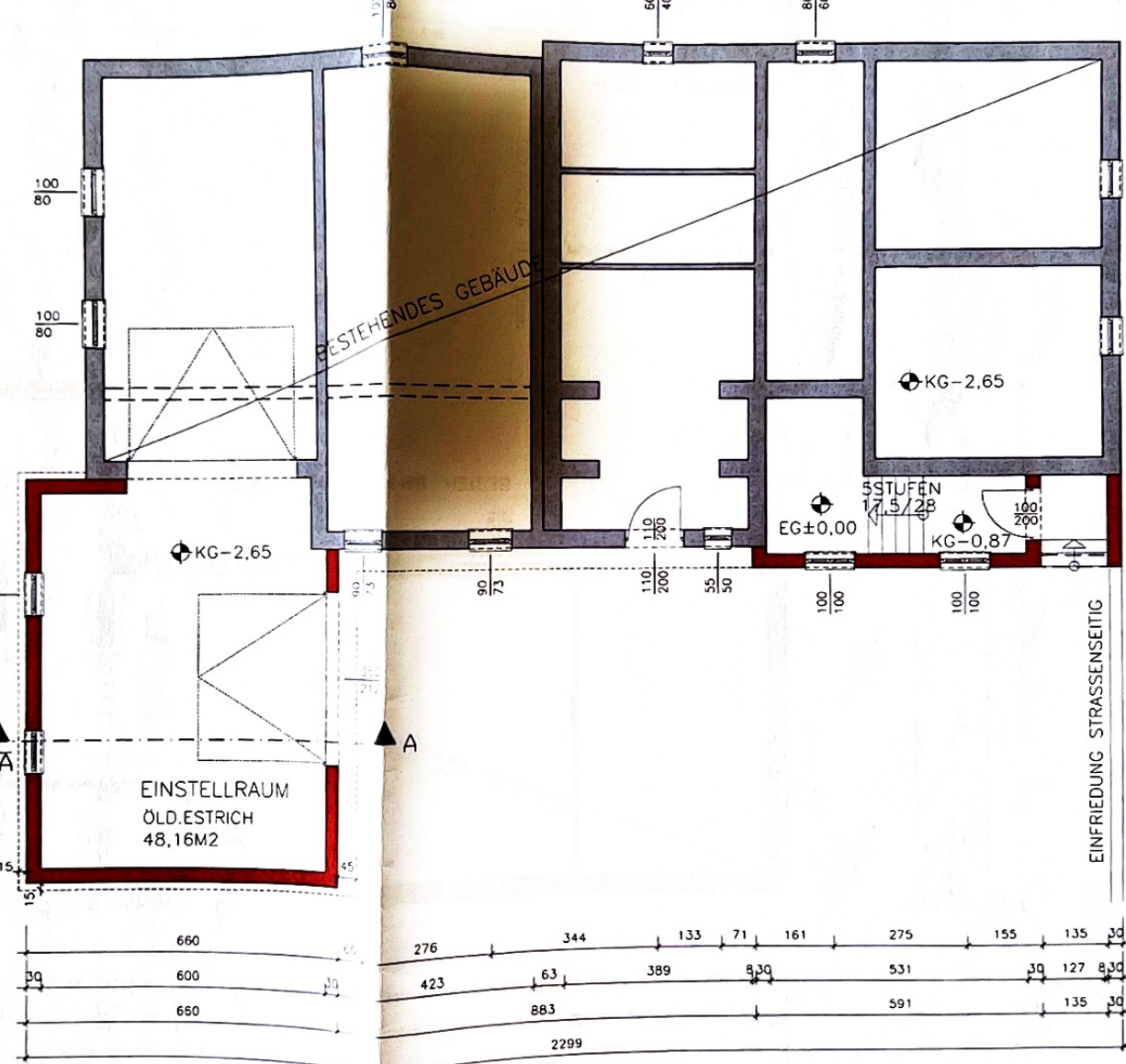
GRUNDRISS KELLERGESCHOSS
