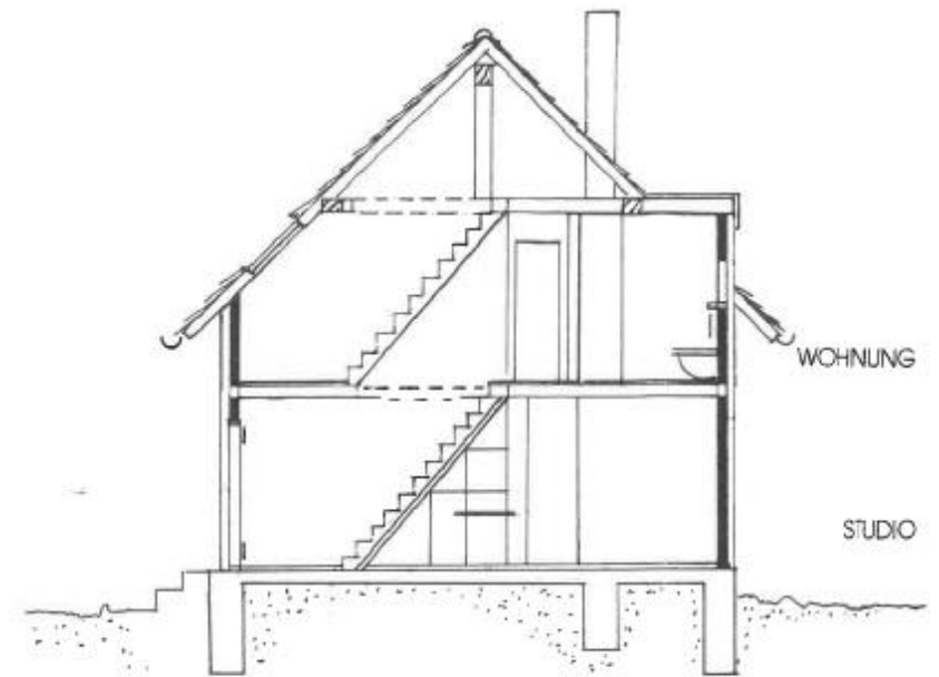
SCHNITT M 1 : 100
