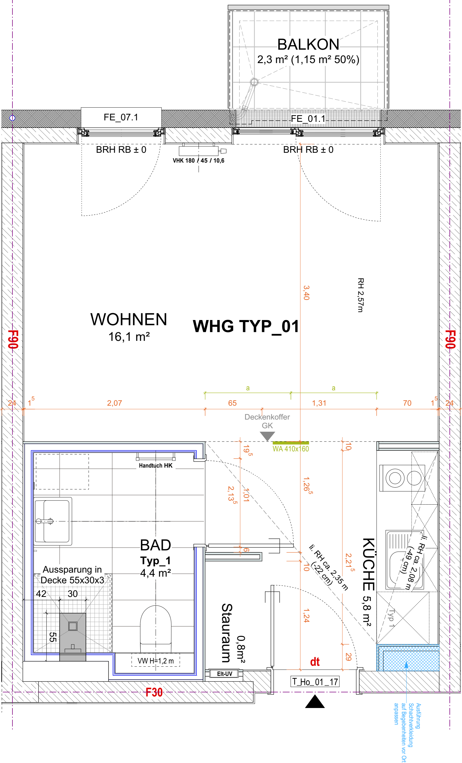
Grundriss 1.-3.OG
