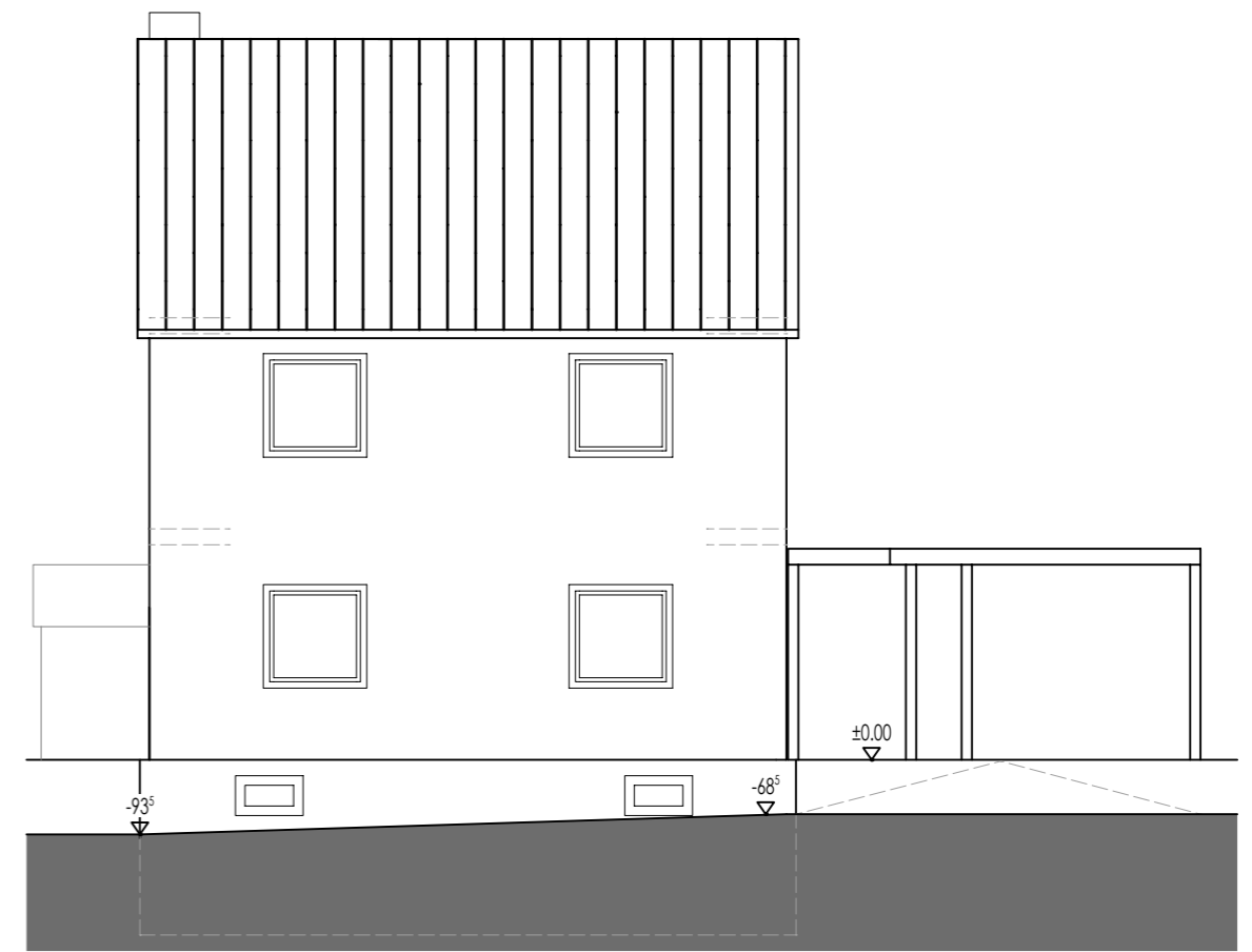
STRASSENANSICHT
